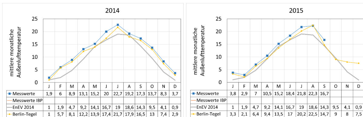
BILD 7-4 GEMESSENE MONATLICHE AUßENLUFTTEMPERATUREN IN DER HINTERLÜFTUNGSEBENE DER NNO-AUßENWAND VON 2014 BIS 2015 UND BEZUG ZU DEN DATEN DER ENEV 2014 SOWIE DER WETTERSTATION BERLIN-TEGEL
