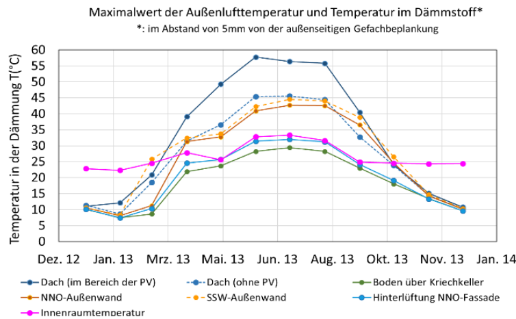
BILD 7-37 MONATLICHE MAXIMALWERTE DER GEMESSENEN TEMPERATUREN INNERHALB DER GEFACHDÄMMUNG DER AUßENBAUTEILE AUßENWAND, BODEN UND DACH MIT 5MM ABSTAND ZUR AUßENSEITIGEN GEFACHBEPLANKUNG FÜR 2013
