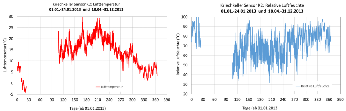
BILD 7-6 GEMESSENE TEMPERATUREN UND RELATIVE LUFTFEUCHTEN IM KRIECHKELLER VON 2013
