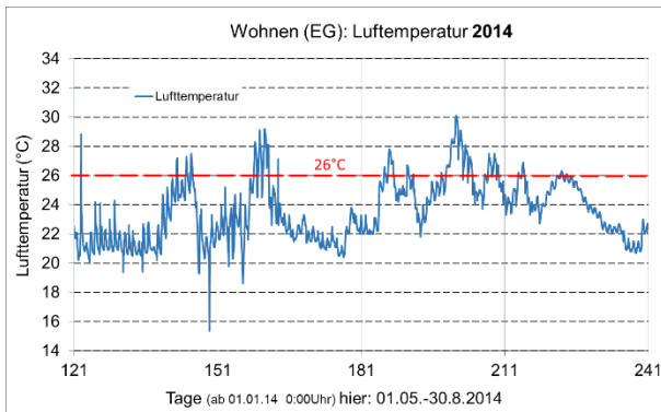
BILD 7-12 GEMESSENE RAUMLUFTTEMPERATUREN IM WOHNRAUM IN 2014: VOM 01. 05.-30.08.14 UND VOM 18.07.-25.07.14
