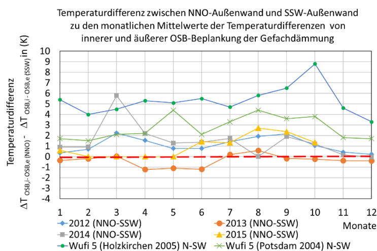
BILD 7-19 TEMPERATURDIFFERENZ ZWISCHEN NNO-AUßENWAND UND SSW-AUßENWAND ZU DEN MONATLICHEN MITTELWERTEN DER TEMPERATURDIFFERENZEN VON ÄUßEREN UND INNERER OSB-BEPLANKUNG DER GEFACHDÄMMUNG \Delta T_{OSB,i - OSB,e (NNO)} - \Delta T_{OSB,i - OSB,e (SSW)}
