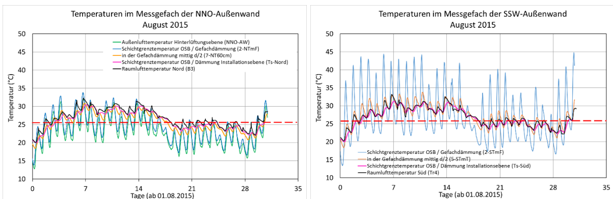
BILD 7-26 GEMESSENE TEMPERATUREN ÜBER DEN QUERSCHNITT DER NNO- UND SSW-AUßENWAND IM AUGUST 2015
