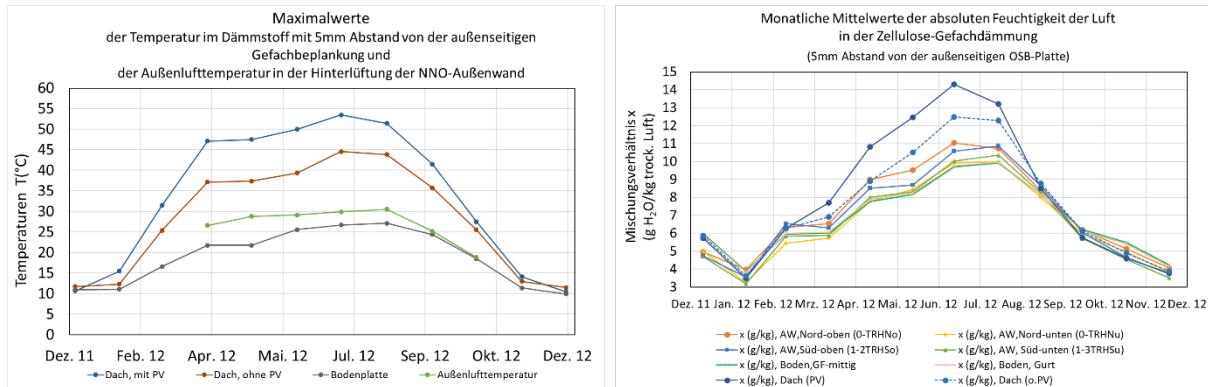
BILD 7-51 MONATLICHE MITTELWERTE GEMESSENER MAXIMALWERTE DER TEMPERATUR IM DÄMMSTOFF IM ABSTAND VON 5MM VON DER AUßENSEITIGEN GEFACHBEPLANKUNG DER AUßENBAUTEILE SOWIE DER MONATLICHEN MITTELWERTE DER ABSOLUTEN FEUCHTIGKEIT IN DER LUFT DER ZELLULOSE-GEFACHDÄMMUNG FÜR 2012
