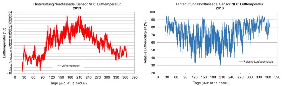
BILD 9-29 GEMESSENE TEMPERATUREN UND RELATIVE LUFTFEUCHTEN IN DER HINTERLÜFTUNGSEBENE DER NNO-AUßENWAND VON 2013
