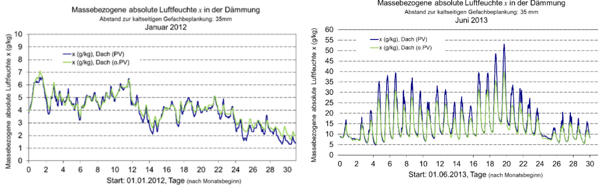
BILD 9-61 MASSEBEZOGENE ABSOLUTE LUFTFEUCHTE IN DER GEFACHDÄMMUNG DES DACHES IM BEREICH DER PV-ELEMENTE UND AUßERHALB DAVON IM JANUAR 2012 UND JUNI 2013
