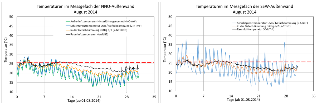
BILD 7-24 GEMESSENE TEMPERATUREN ÜBER DEN QUERSCHNITT DER NNO- UND SSW-AUßENWAND IM AUGUST 2014
