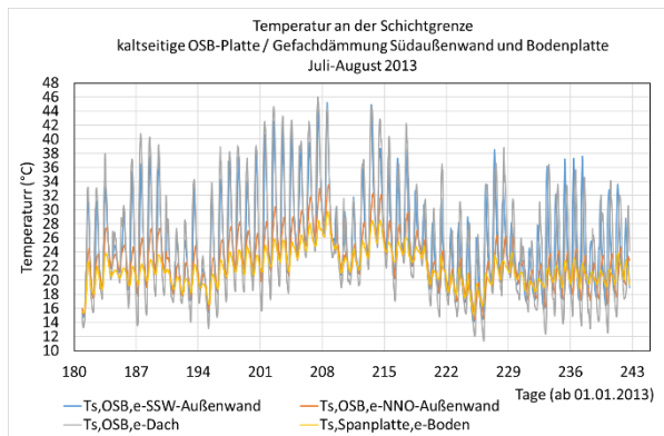
BILD 7-34 GEMESSENE TEMPERATUREN AN DER SCHICHTGRENZE DER AUßENSEITIGEN GEFACHBEPLANKUNG DER NNO-AUßENWAND, SSW-AUßENWAND, IM DACH (AUßERHALB DES BEREICHES DER PV-ELEMENTE) UND IN DER BODENPLATTE ÜBER DEM KRIECKELLER VON JULI BIS AUGUST 2013
