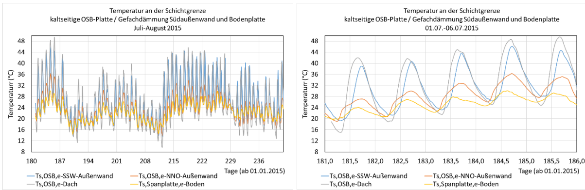
BILD 7-36 GEMESSENE TEMPERATUREN AN DER SCHICHTGRENZE DER AUßENSEITIGEN GEFACHBEPLANKUNG DER NNO-AUßENWAND, SSW-AUßENWAND, IM DACH (AUßERHALB DES BEREICHES DER PV-ELEMENTE) UND IN DER BODENPLATTE ÜBER DEM KRIECKELLER VON JULI BIS AUGUST 2015
