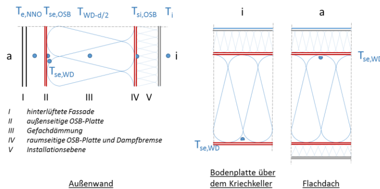
BILD 7-20 LAGE DER TEMPERATURSENSOREN FÜR DIE BEWERTUNG DES SOMMERLICHEN WÄRMESCHUTZES
