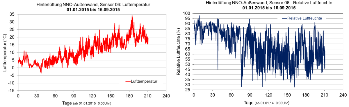
BILD 9-31 GEMESSENE TEMPERATUREN UND RELATIVE LUFTFEUCHTEN IN DER HINTERLÜFTUNGSEBENE DER NNO-AUßENWAND VON 2015
