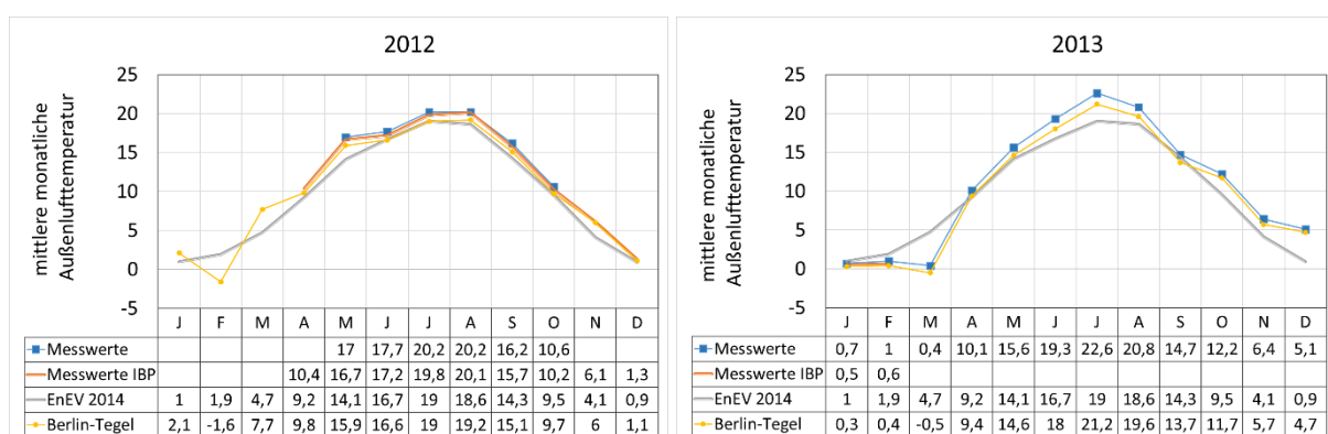
BILD 7-3 GEMESSENE MONATLICHE AUßENLUFTTEMPERATUREN IN DER HINTERLÜFTUNGSEBENE DER NNO-AUßENWAND VON 2012 BIS 2013 UND BEZUG ZU DEN DATEN DER ENEV 2014 SOWIE DER WETTERSTATION BERLIN-TEGEL
