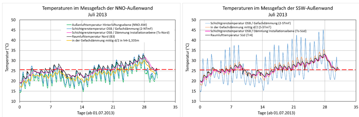
BILD 7-21 GEMESSENE TEMPERATUREN ÜBER DEN QUERSCHNITT DER NNO- UND SSW-AUßENWAND IM JULI 2013
