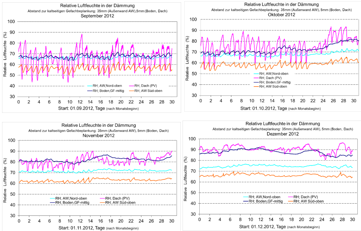
BILD 9-50 RELATIVE LUFTFEUCHTEN IN DER GEFACHDÄMMUNG DER AUßENWAND, DER BODENPATTE UND DES DACHES VON SEPTEMBER BIS DEZEMBER 2012
