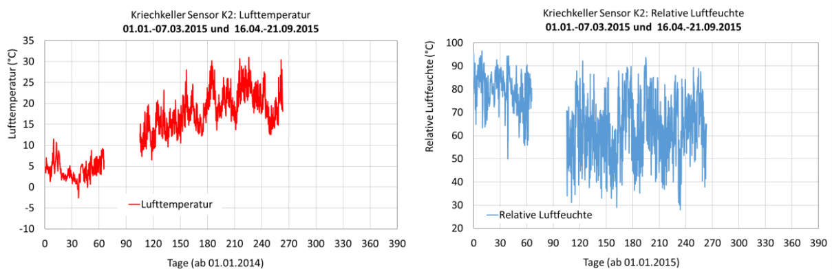
BILD 7-8 GEMESSENE TEMPERATUREN UND RELATIVE LUFTFEUCHTEN IM KRIECHKELLER VON 2015
