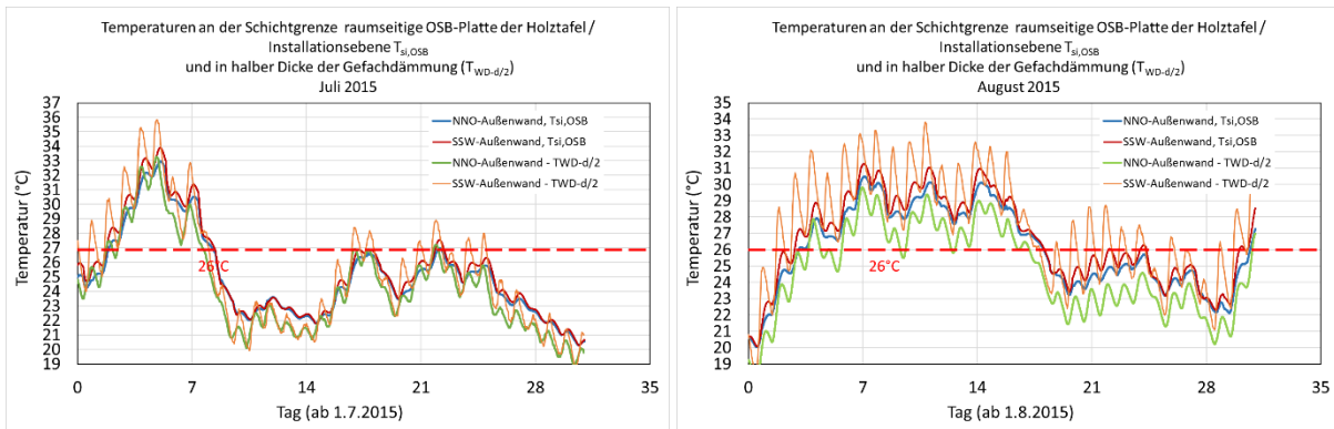
BILD 7-32 TEMPERATUREN INNERHALB DER GEFACHDÄMMUNG DER AUßENBAUTEILE, GEMESSEN IM ABSTAND VON 5MM ZUR AUßENSEITIGEN GEFACHBEPLANKUNG: JULI UND AUGUST 2015
