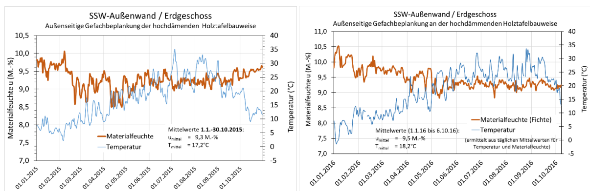
BILD 9-37 GEMESSENE MATERIALFEUCHTEN UND TEMPERATUREN ALS TÄGLICHE MITTELWERTE IN DER AUßENSEITIGEN GEFACHBEPLANKUNG DER SSW-AUßENWAND / ERDGESCHOSS FÜR 2015 UND VOM 1.1.-06.10. 2016
