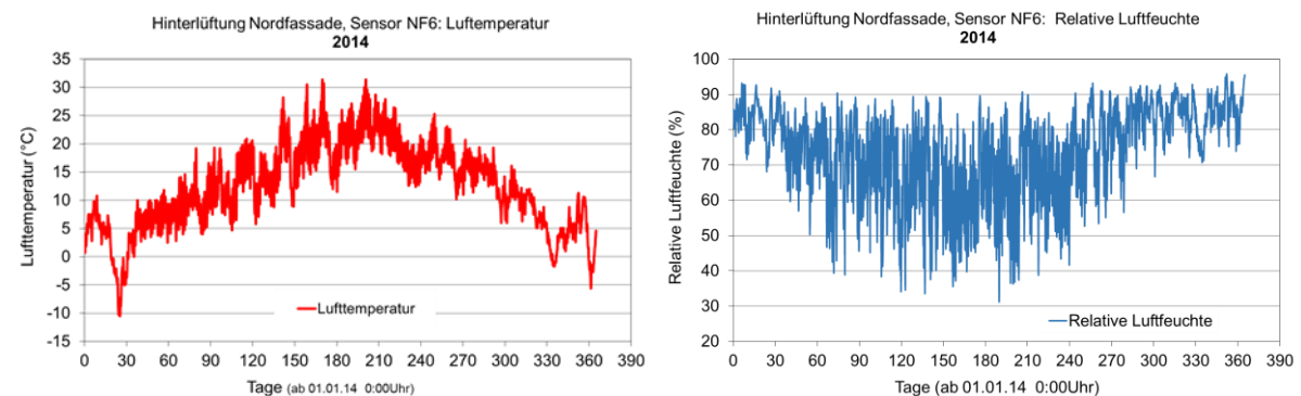
BILD 9-30 GEMESSENE TEMPERATUREN UND RELATIVE LUFTFEUCHTEN IN DER HINTERLÜFTUNGSEBENE DER NNO-AUßENWAND VON 2014
