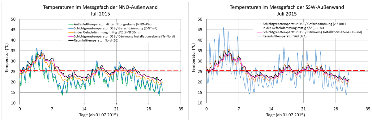
BILD 7-25 GEMESSENE TEMPERATUREN ÜBER DEN QUERSCHNITT DER NNO- UND SSW-AUßENWAND IM JULI 2015
