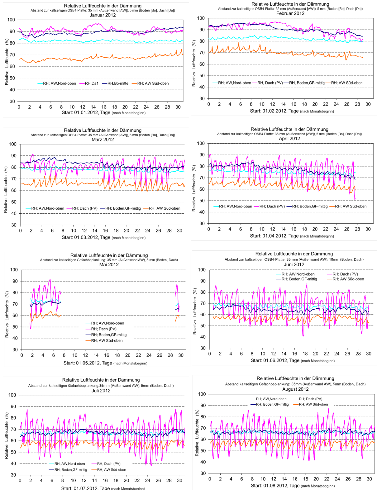
BILD 9-49 RELATIVE LUFTFEUCHTEN IN DER GEFACHDÄMMUNG DER AUßENWAND, DER BODENPATTE UND DES DACHES VON JANUAR BIS AUGUST 2012
