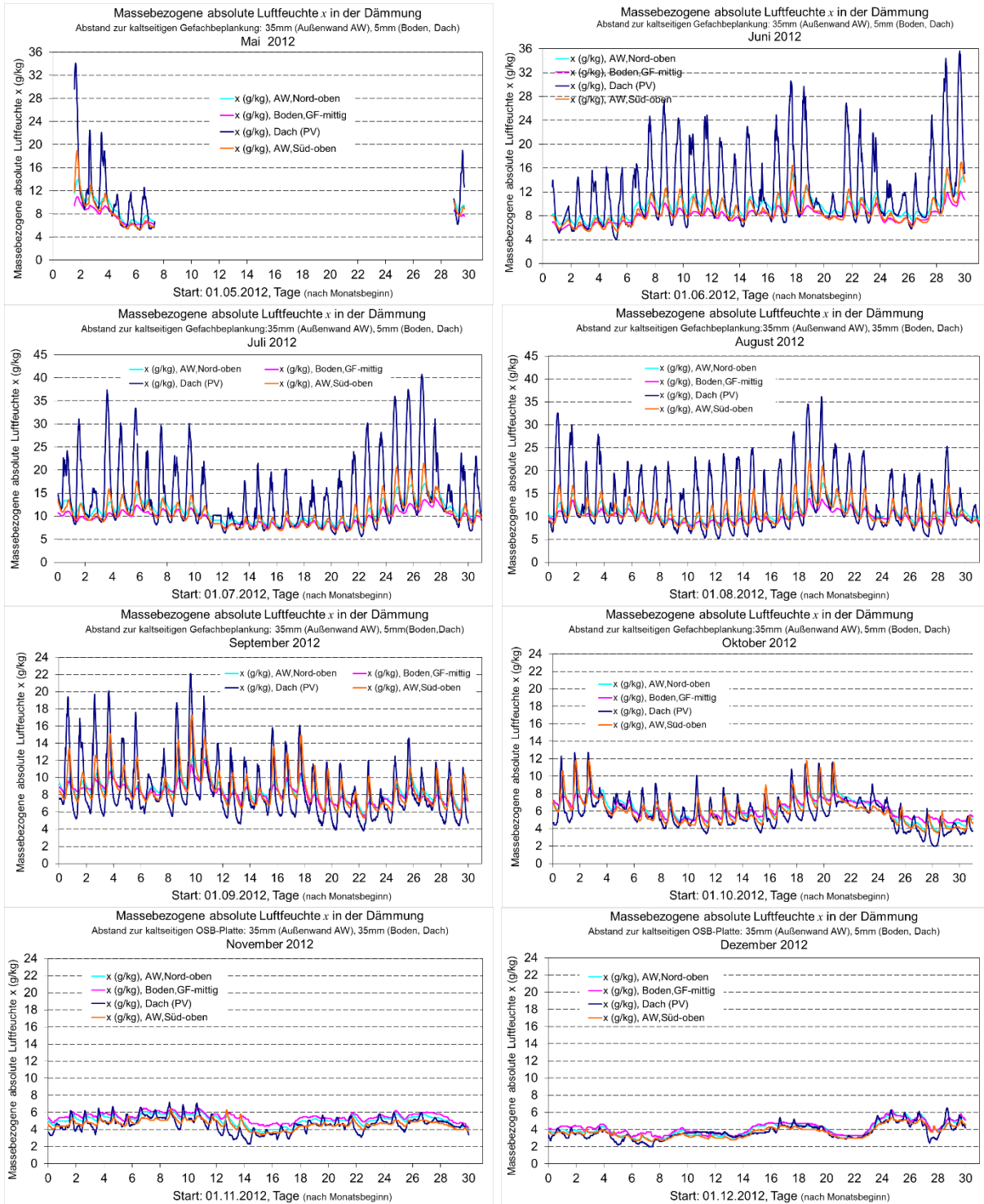
BILD 9-60 MASSEBEZOGENE ABSOLUTE LUFTFEUCHTE IN DER GEFACHDÄMMUNG DER AUßENWAND, DER BODENPATTE UND DES DACHES VON MAI 2012 BIS DEZEMBER 2012
