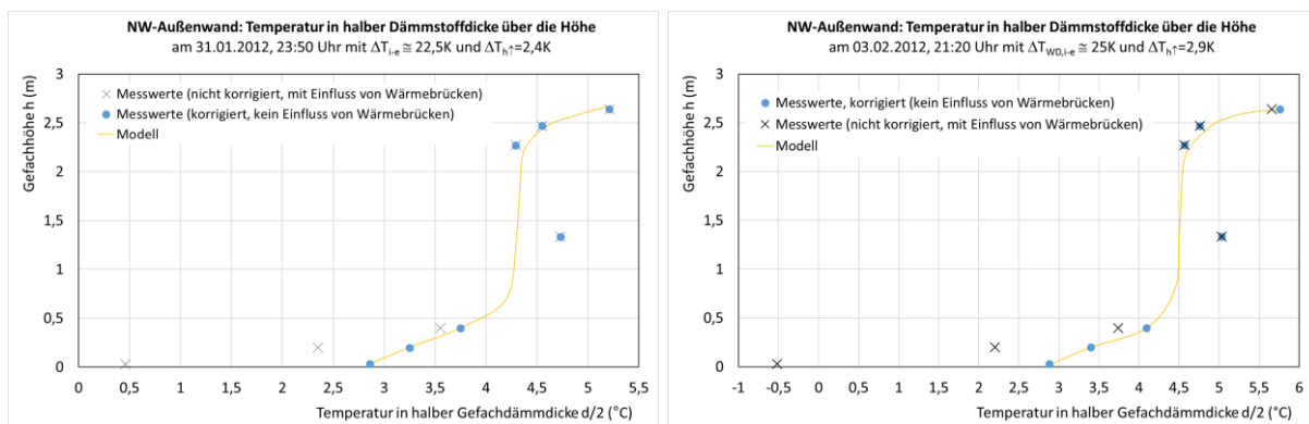
BILD 7-45 TEMPERATUREN IN HALBER GEFACHDÄMMDICKE IN VERSCHIEDENEN HÖHEN FÜR DIE DARSTELLUNG EINES FÜR NATÜRLICHE KONVEKTION TYPISCHEN TEMPERATURVERLAUFES ÜBER DIE HÖHE: MESSWERTE VOM 31.01.2012 UND VOM 03.02.2012 SOWIE DARSTELLUNG DES EINFLUSSES VON WÄRMEBRÜCKEN AUS WÄRMELEITUNG
