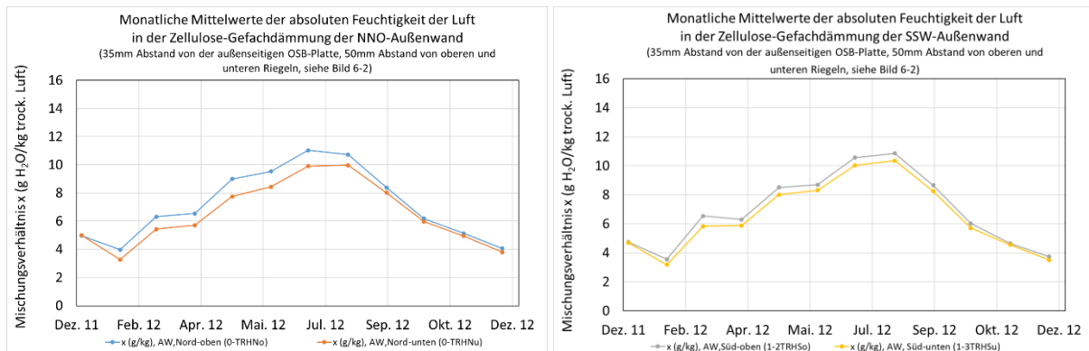
BILD 7-47 GEMESSENE MONATLICHE MITTELWERTE DER ABSOLUTEN FEUCHTIGKEIT DER LUFT IM DÄMMSTOFF IM ABSTAND VON 35MM VON DER AUßENSEITIGEN GEFACHBEPLANKUNG DER NNO-AUßENWAND UND DER SSW-AUßENWAND FÜR 2012
