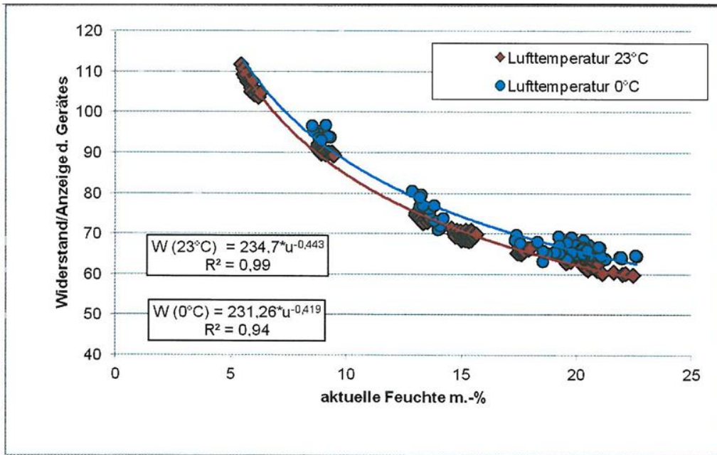
BILD 9-12 EXPERIMENTELL ERMITTELTE BEZIEHUNG ZWISCHEN DEM ELEKTRISCHEN WIDERSTAND UND DER MATERIALFEUCHTE AN OSB BEI TEMPERATUREN VON 23°C UND VON 0°C
