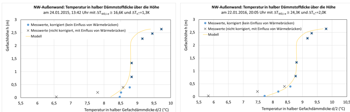
BILD 7-46 TEMPERATUREN IN HALBER GEFACHDÄMMDICKE IN VERSCHIEDENEN HÖHEN FÜR DIE DARSTELLUNG EINES FÜR NATÜRLICHE KONVEKTION TYPISCHEN TEMPERATURVERLAUFES ÜBER DIE HÖHE: MESSWERTE VOM 24.01.2015 UND VOM 22.01.2016 SOWIE DARSTELLUNG DES EINFLUSSES VON WÄRMEBRÜCKEN AUS WÄRMELEITUNG
