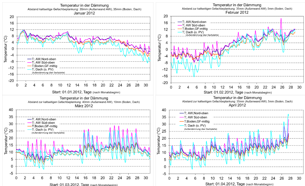
BILD 9-55 TEMPERATUR IN DER GEFACHDÄMMUNG DER AUßENWAND, DER BODENPATTE UND DES DACHES VON JANUAR 2012 BIS APRIL 2012 (ZUZUORDNEN DER RELATIVEN LUFTFEUCHTE AUS ABSCHNITT 9.4.3)
