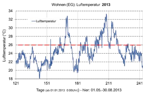
BILD 7-11 GEMESSENE RAUMLUFTTEMPERATUREN IM WOHNRAUM IN 2013: VOM 01. 05.-31.08.13 UND VOM 18.06.-25.06.13
