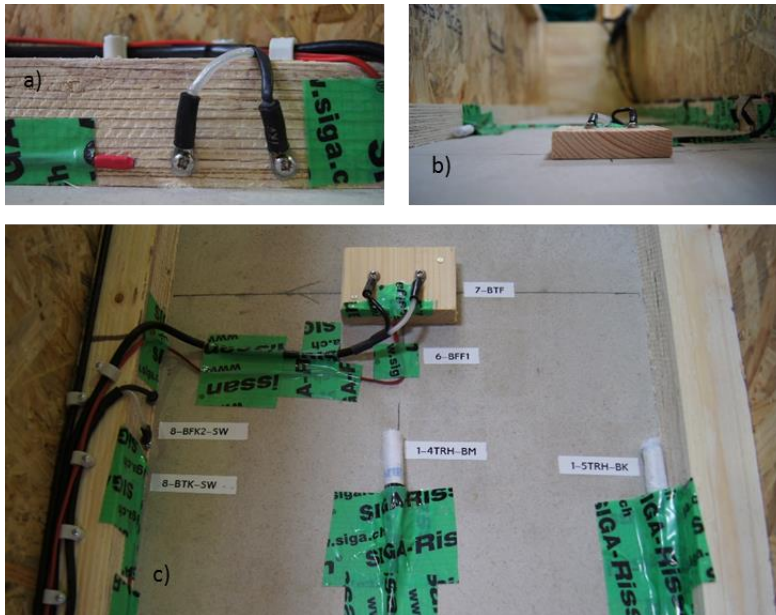
BILD 6-7 FOTOS ZUR BAUWEISE UND ANORDNUNG DER MESSFÜHLER IM BODENGEFACH: A) EINSCHLAGEELEKTRODEN IN KERTO-GURT UND ZUGEHÖRIGER TEMPERATURFÜHLER ZUR TEMPERATURKOMPENSATION DER MATERIALFEUCHTE, B) EINSCHLAGEELEKTRODEN IN FICHTENHOLZ, C) ÜBERBLICK ÜBER DIE LAGE DER MESSFÜHLER
