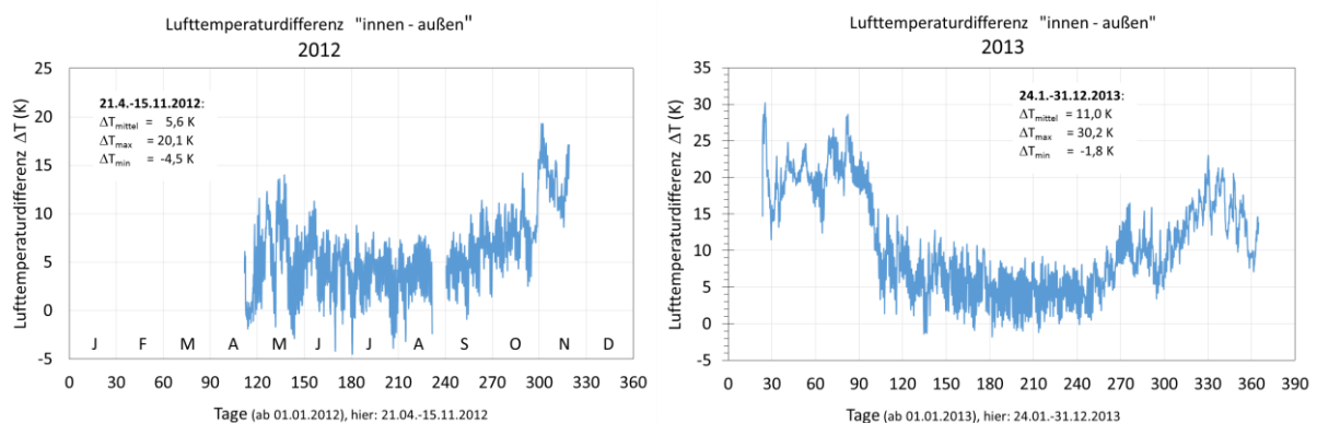
BILD 7-15 LUFTTEMPERATURDIFFERENZEN AUS DEN GEMESSENEN TEMPERATUREN VOM INNENRAUM ( T_{r4} ) UND DER HINTERLÜFTUNGSEBENE DER NNO-AUßENWAND FÜR 2012 UND 2013
