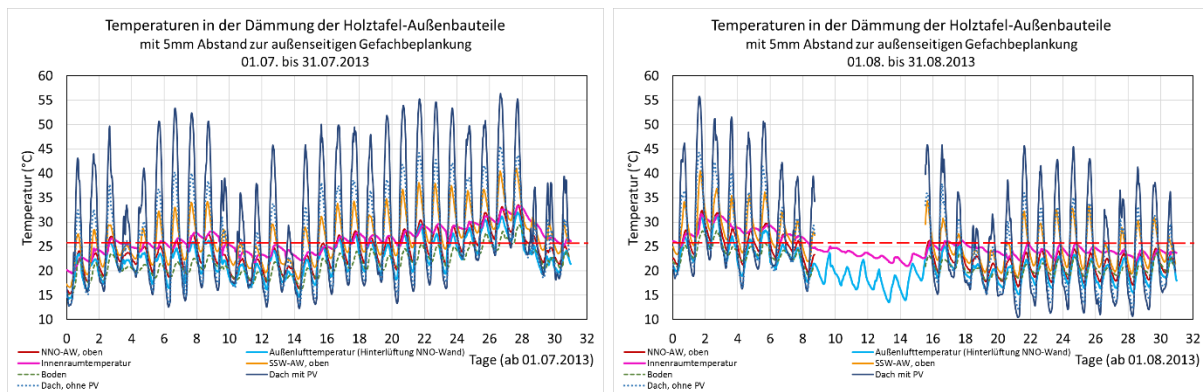
BILD 7-29 GEMESSENE TEMPERATUREN NAHE DEN SCHICHTGRENZEN DER AUßENSEITIGEN OSB-PLATTEN DER NNO- UND SSW-AUßENWAND, DER BODENPLATTE (ÜBER DEM KRIECKELLER: ZEMENTGEBUNDENE SPANPLATTE) UND IM DACH IM JULI 2015
