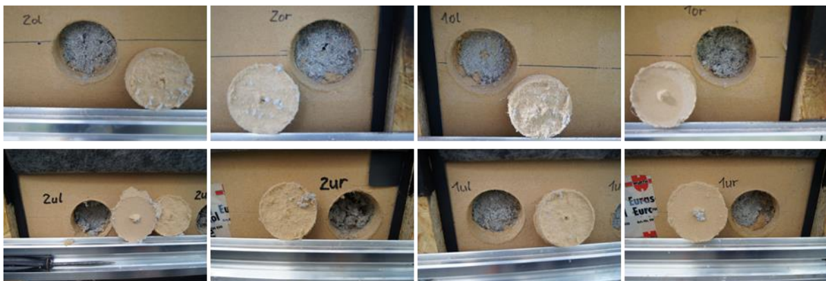
BILD 9-16 ZUSTAND DER SCHICHTGRENZE GEFACHDÄMMUNG / AUßENSEITIGE GEFACHBEPLANKUNG AN GEFACH 1 UND 2 AM 27.04.2012
