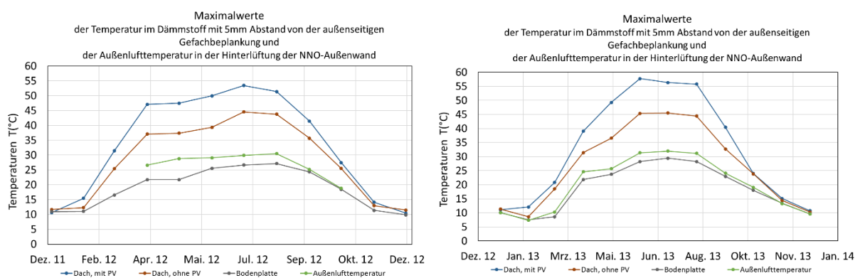
BILD 7-39 GEMESSENE MAXIMALWERTE DER TEMPERATUR IM DÄMMSTOFF IM ABSTAND VON 5MM VON DER AUßENSEITIGEN GEFACHBEPLANKUNG IM DACH, IM UND AUßERHALB DES BEREICHES DER PV-ELEMENTE, IN DER BODENPLATTE SOWIE DIE AUßENLUFTTEMPERATUR FÜR 2012 UND 2013
