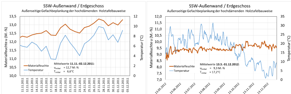
BILD 9-35 GEMESSENE MATERIALFEUCHTEN UND TEMPERATUREN ALS TÄGLICHE MITTELWERTE IN DER AUßENSEITIGEN GEFACHBEPLANKUNG DER SSW-AUßENWAND / ERDGESCHOSS FÜR DEZEMBER 2011 (EINBAU) UND FÜR 2012
