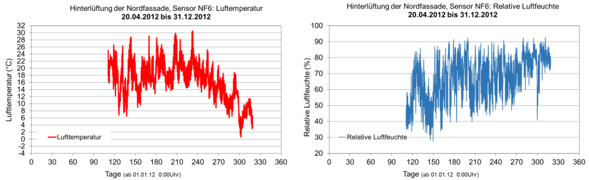
BILD 9-28 GEMESSENE TEMPERATUREN UND RELATIVE LUFTFEUCHTEN IN DER HINTERLÜFTUNGSEBENE DER NNO-AUßENWAND VON 2012
