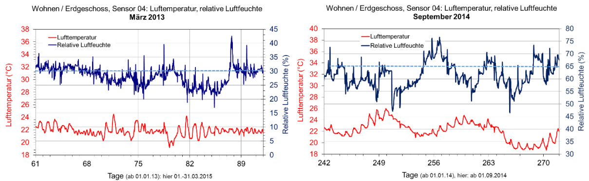
BILD 7-14 GEMESSENE INNENLUFTTEMPERATUREN UND RELATIVE LUFTFEUCHTEN IM WOHNRAUM FÜR MÄRZ 2015 UND FÜR SEPTEMBER 2014
