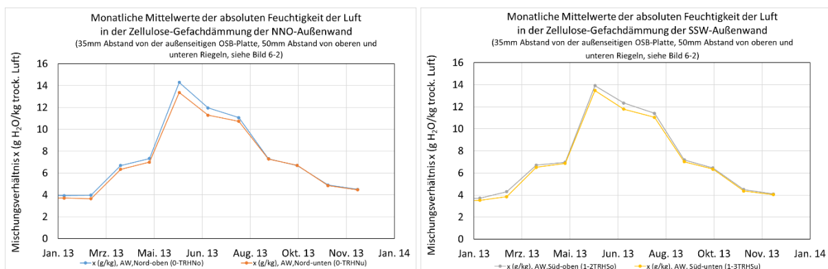
BILD 7-48 GEMESSENE MONATLICHE MITTELWERTE DER ABSOLUTEN FEUCHTIGKEIT DER LUFT IM DÄMMSTOFF IM ABSTAND VON 35MM VON DER AUßENSEITIGEN GEFACHBEPLANKUNG DER NNO-AUßENWAND UND DER SSW-AUßENWAND FÜR 2013
