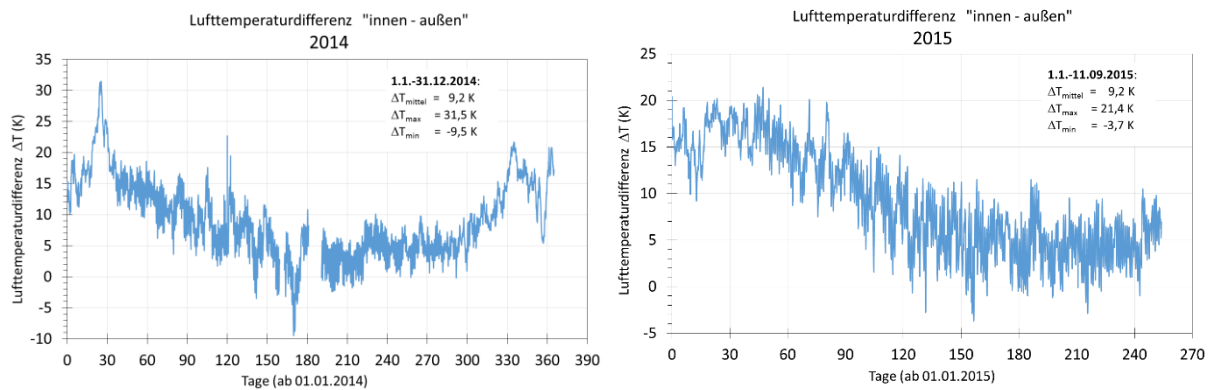
BILD 7-16 LUFTTEMPERATURDIFFERENZEN AUS DEN GEMESSENEN TEMPERATUREN VOM INNENRAUM (Tr4) UND DER HINTERLÜFTUNGSEBENE DER NNO-AUßENWAND FÜR 2014 UND 2015
