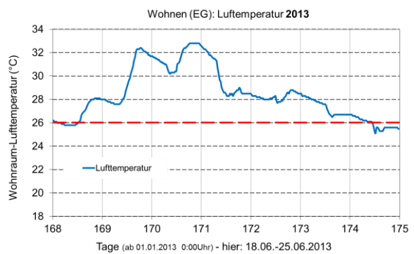
BILD 7-11 GEMESSENE RAUMLUFTTEMPERATUREN IM WOHNRAUM IN 2013: VOM 01. 05.-31.08.13 UND VOM 18.06.-25.06.13
