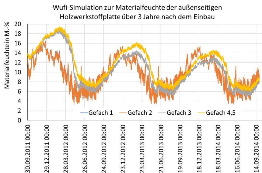
BILD 7-43 ERGEBNISSE VON SIMULATIONSRECHNUNGEN MIT WUFI PRO 5.0 ZUR MATERIALFEUCHTE DER AUßENSEITIGEN HOLZTAFELBEPLANKUNGEN MIT OSB4 (GEFACHE 3, 4 UND 5) UND EINER DIFFUSIONSOFFENEN HOLZWEICHFASERPLATTE (GEFACHE 1 UND 2) BEI UNTERSCHIEDLICHEN s_{di} - UND s_{de} -WERTEN DER AUßENWANDGEFACHE
