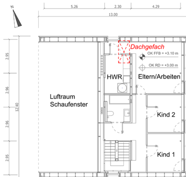
Grundriss Obergeschoss (Entwurf / Architekturzeichnung Werner Sobeck Engineering & Design)
