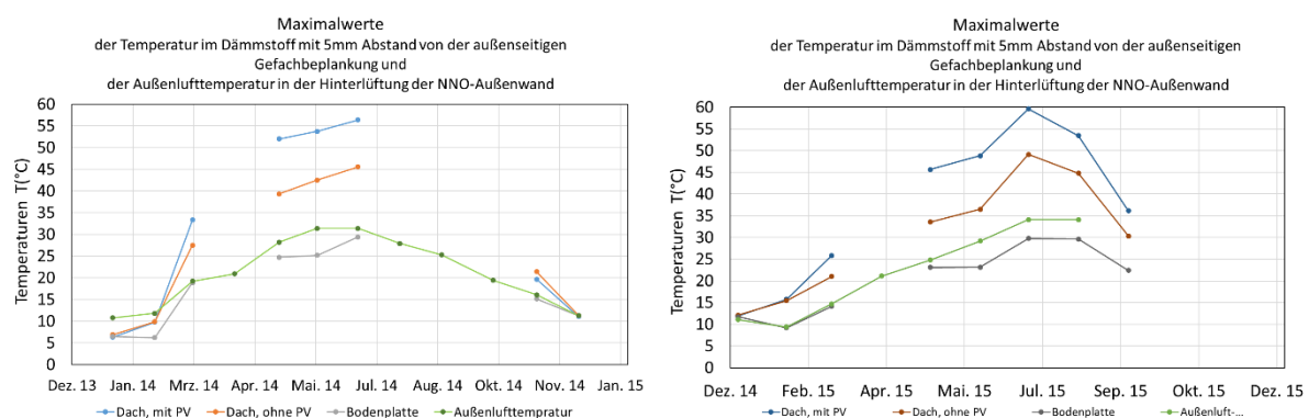
BILD 7-40 GEMESSENE MAXIMALWERTE DER TEMPERATUR IM DÄMMSTOFF IM ABSTAND VON 5MM VON DER AUßENSEITIGEN GEFACHBEPLANKUNG IM DACH, IM UND AUßERHALB DES BEREICHES DER PV-ELEMENTE, IN DER BODENPLATTE SOWIE DIE AUßENLUFTTEMPERATUR FÜR 2014 UND 2015
