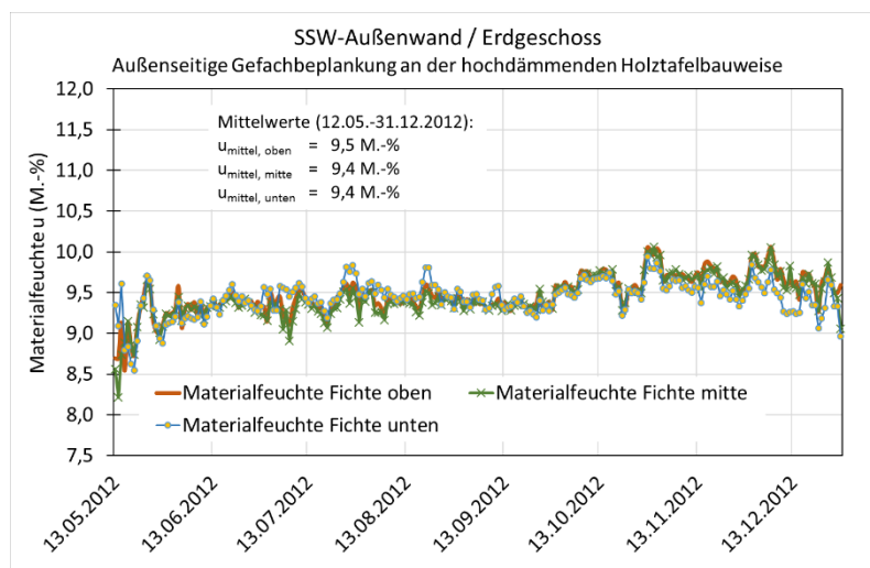
BILD 7-42 MESSWERTE ZUR MATERIALFEUCHTE IN DER AUßENSEITIGEN OSB-GEFACHBEPLANKUNG DER SSW-AUßENWAND (EG) VON 2012
