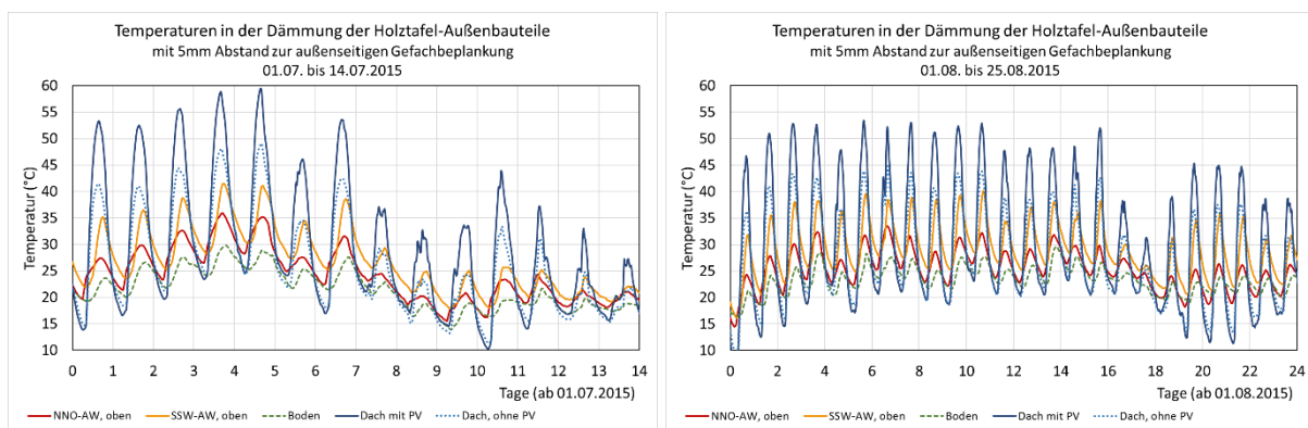
BILD 7-30 GEMESSENE TEMPERATUREN NAHE DEN SCHICHTGRENZEN DER AUßENSEITIGEN OSB-PLATTEN DER NNO- UND SSW-AUßENWAND, DER BODENPLATTE (ÜBER DEM KRIECKELLER: ZEMENTGEBUNDENE SPANPLATTE) UND IM DACH IM JULI 2015
