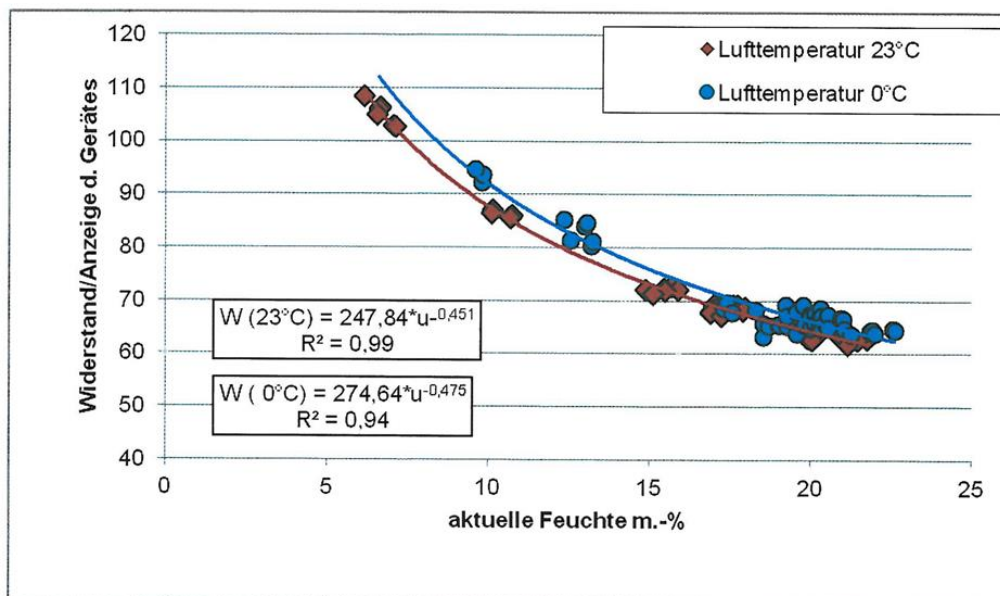
BILD 9-11 EXPERIMENTELL ERMITTELTE BEZIEHUNG ZWISCHEN DEM ELEKTRISCHEN WIDERSTAND UND DER MATERIALFEUCHTE AN FICHTE (QUER ZUR FASER) BEI TEMPERATUREN VON 23°C UND VON 0°C
