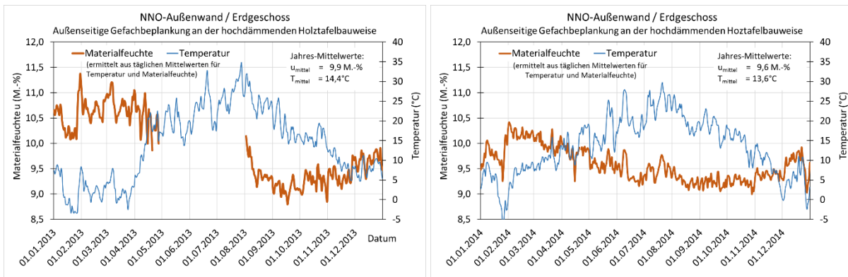
BILD 9-33 GEMESSENE MATERIALFEUCHTEN UND TEMPERATUREN ALS TÄGLICHE MITTELWERTE IN DER AUßENSEITIGEN GEFACHBEPLANKUNG DER NNO-AUßENWAND / ERDGESCHOSS FÜR 2013 UND 2014
