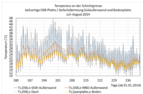
BILD 7-35 GEMESSENE TEMPERATUREN AN DER SCHICHTGRENZE DER AUßENSEITIGEN GEFACHBEPLANKUNG DER NNO-AUßENWAND, SSW-AUßENWAND, IM DACH (AUßERHALB DES BEREICHES DER PV-ELEMENTE) UND IN DER BODENPLATTE ÜBER DEM KRIECKELLER VON JULI BIS AUGUST 2014
