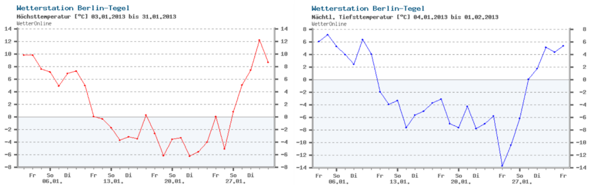
BILD 9-24 HÖCHST- UND TIEFTEMPERATUREN VOR UND WÄHREND DER ORTSBESICHTIGUNG AM 24.01.2013 (QUELLE: WWW.WETTERONLINE.DE)
