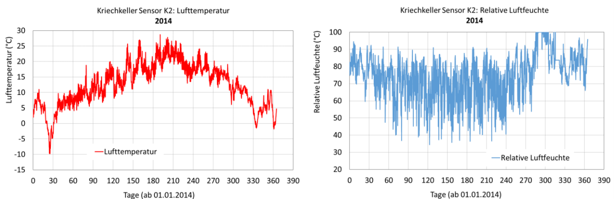
BILD 7-7 GEMESSENE TEMPERATUREN UND RELATIVE LUFTFEUCHTEN IM KRIECHKELLER VON 2014
