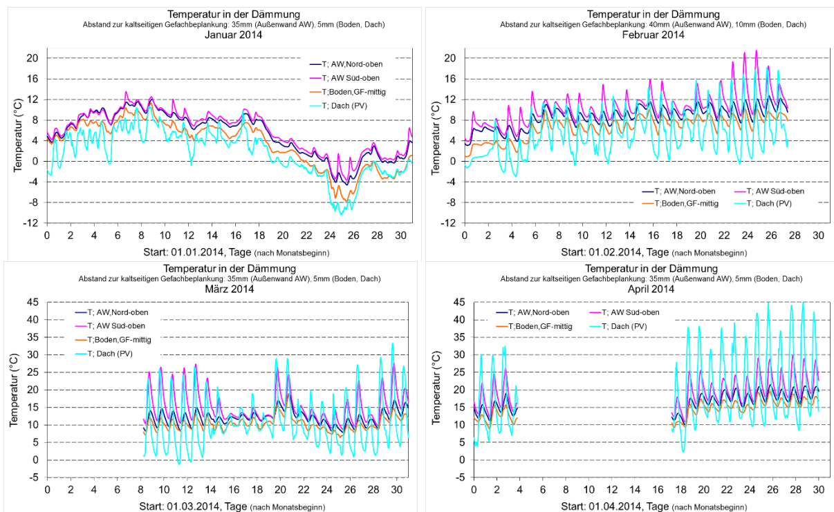
BILD 9-57 TEMPERATUR IN DER GEFACHDÄMMUNG DER ÄUßENWAND, DER BODENPATTE UND DES DACHES VON JANUAR 2014 BIS APRIL 2014 (ZUZUORDNEN DER RELATIVEN LUFTFEUCHTE AUS ABSCHNITT 9.4.3)
