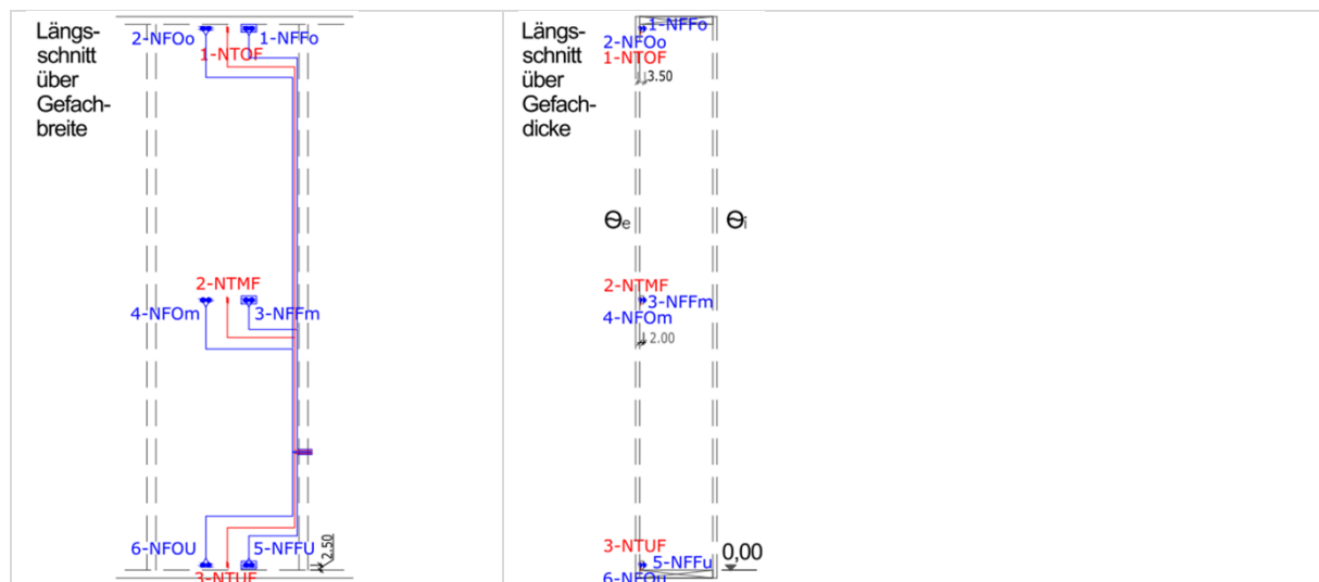
BILD 6-6 ÜBERSICHTSZEICHNUNGEN ZUR ANORDNUNG VON EINSCHLAGEELEKTRODEN IN DIE AUßENSEITIGE OSB-PLATTE UND IN FICHTENHOLZ-ADAPTER VON GEFACH NR. 5 DER NNO-AUßENWAND SOWIE ZUR ANORDNUNG DER ZUGEORDNETEN TEMPERATURFÜHLER ZWECKS TEMPERATUR-KOMPENSATION DER WIDERSTANDSMESSUNG
