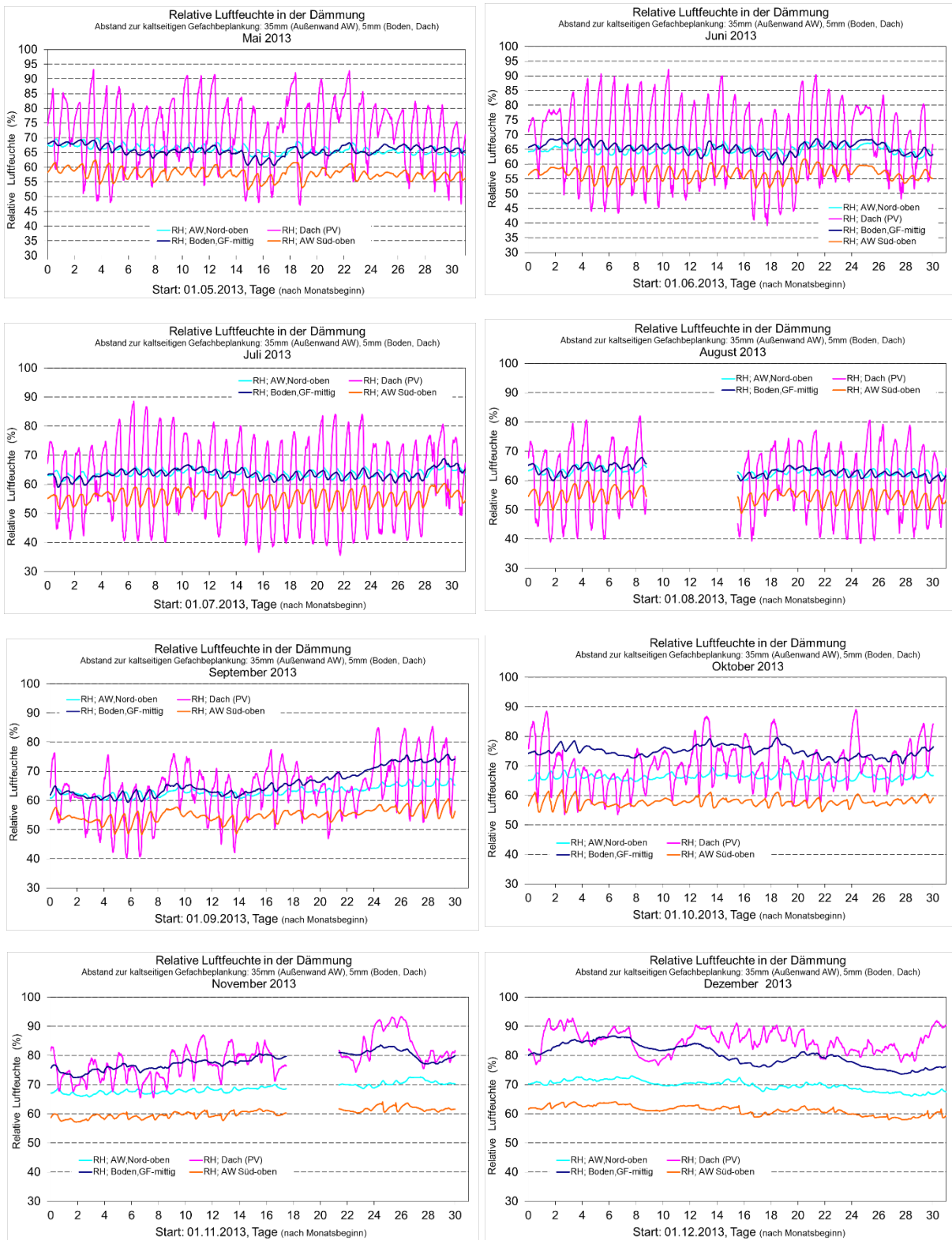
BILD 9-52 RELATIVE LUFTFEUCHTEN IN DER GEFACHDÄMMUNG DER AUßENWAND, DER BODENPATTE UND DES DACHES VON MAI BIS DEZEMBER 2013
