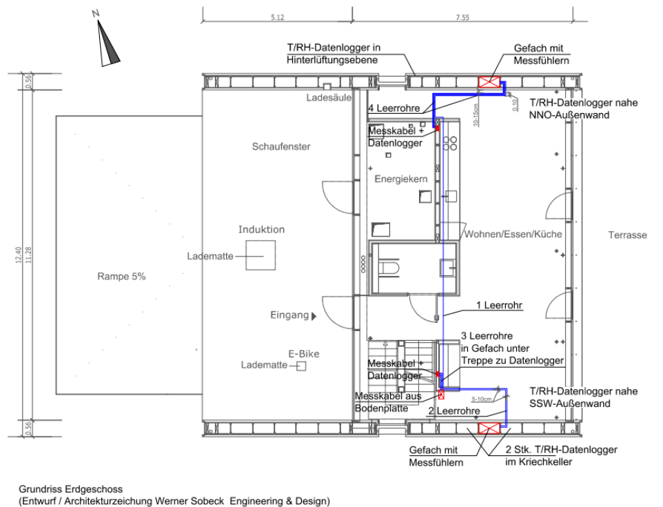
BILD 5-1 ÜBERSICHTSZEICHNUNG ZUR ANORDNUNG VON MESSFÜHLERN IN BAUTEILEN DES ERDGESCHOSSES, DER LAGE DER MESSKABEL IM FUßBODEN ERDGESCHOSS UND DER LAGE DER DATENLOGGER
