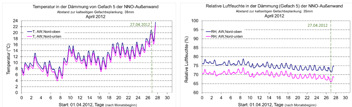
BILD 9-20 TEMPERATUREN UND RELATIVE LUFTFEUCHTEN DER SENSOREN 0-TRHNO UND 1-TRHNU IN DER DÄMMUNG VON GEFACH NUMMER 5 DER NNO-AUßENWAND IM APRIL 2012
