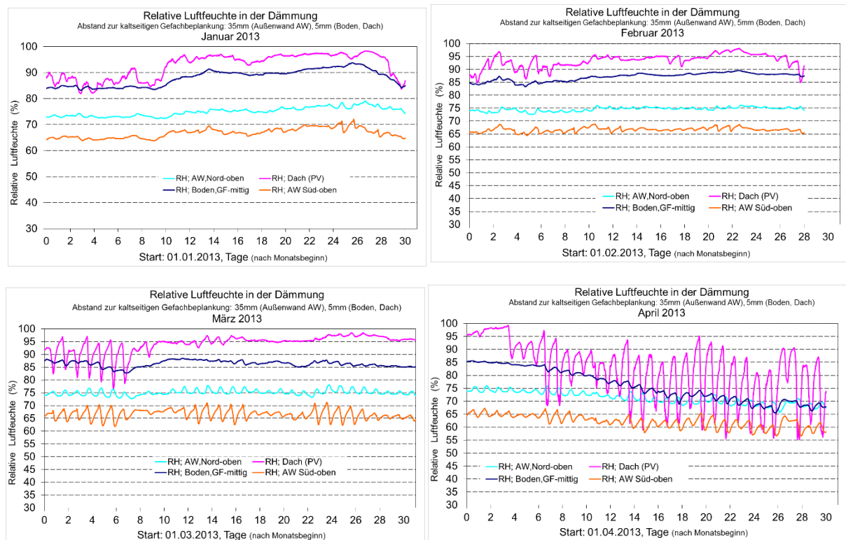
BILD 9-51 RELATIVE LUFTFEUCHTEN IN DER GEFACHDÄMMUNG DER AUßENWAND, DER BODENPATTE UND DES DACHES VON JANUAR BIS APRIL 2013
