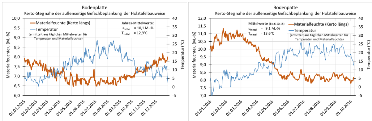
BILD 9-48 GEMESSENE MATERIALFEUCHTEN UND TEMPERATUREN ALS TÄGLICHE MITTELWERTE AN DER AUßENSEITIGEN GEFACHBEPLANKUNG DER HOLZTAFELPLATTE DER BODENPLATTE ÜBER DEM KRIECHKELLER FÜR 2015 UND 2016, MESSWERTE DER SENSOREN 7-BFK1 UND 8-BTK-SW
