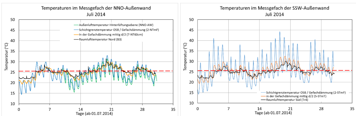
BILD 7-23 GEMESSENE TEMPERATUREN ÜBER DEN QUERSCHNITT DER NNO- UND SSW-AUßENWAND IM JULI 2014
