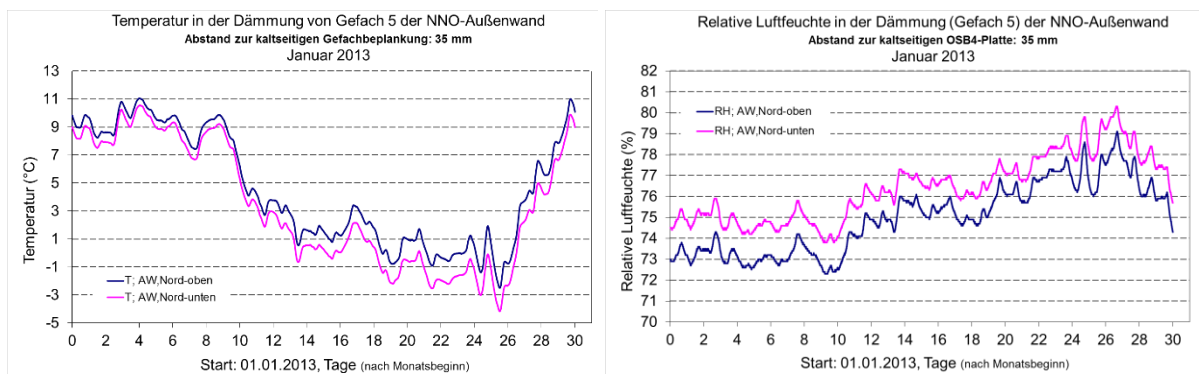
BILD 9-25 TEMPERATUREN UND RELATIVE LUFTFEUCHTEN DER SENSOREN 0-TRHNO UND 1-TRHNU IN DER DÄMMUNG VON GEFACH NUMMER 5 DER NNO-AUßENWAND IM JANUAR 2013
