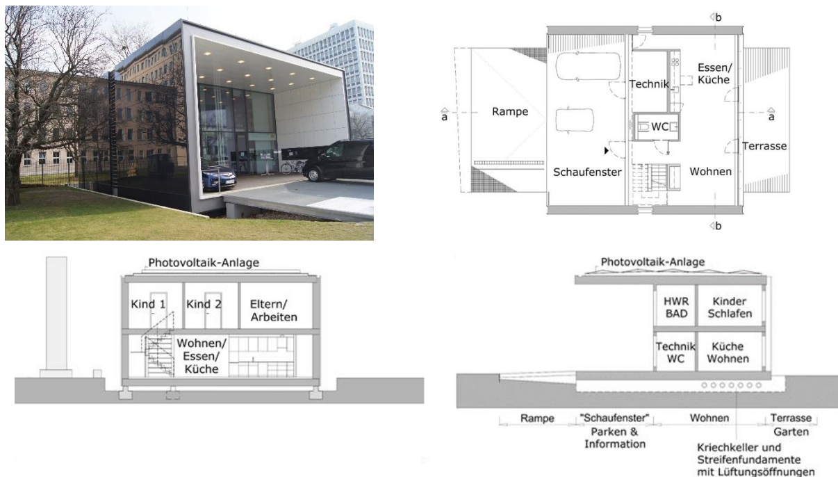
BILD 3-1 DAS „EFFIZIENZHAUS PLUS MIT ELEKTROMOBILITÄT IN BERLIN“ – FOTO UND ÜBERSICHTSZEICHNUNGEN
