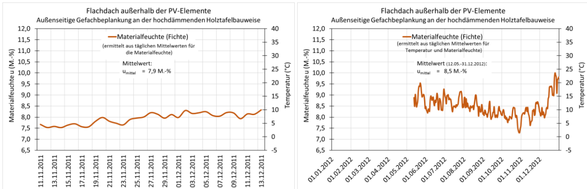
BILD 9-41 GEMESSENE MATERIALFEUCHTEN UND TEMPERATUREN ALS TÄGLICHE MITTELWERTE IN DER AUßENSEITIGEN GEFACHBEPLANKUNG DER HOLZTAFELPLATTE DES FLACHDACHES AUßERHALB DER PV-ELEMENTE FÜR DEZEMBER 2011 (EINBAU) UND FÜR 2012
