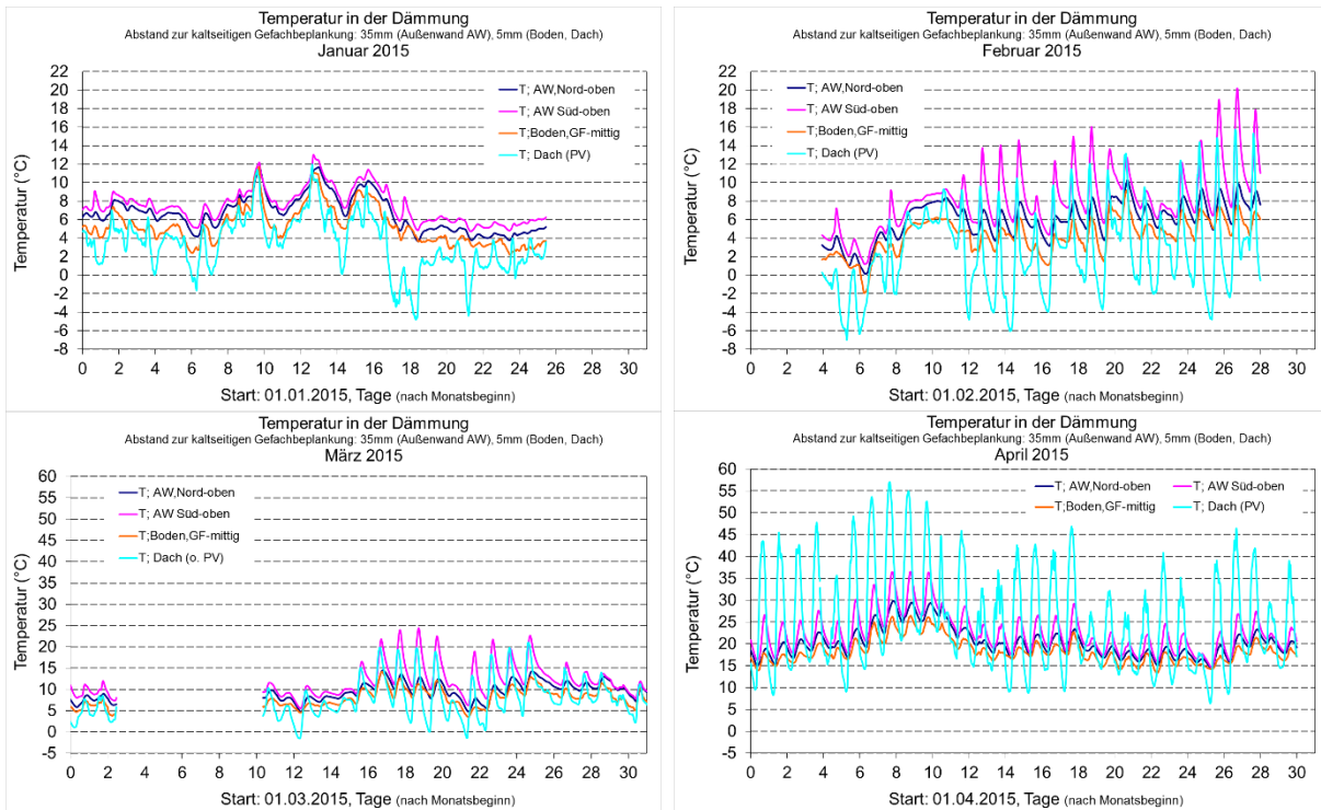
BILD 9-58 TEMPERATUR IN DER GEFACHDÄMMUNG DER AUßENWAND, DER BODENPATTE UND DES DACHES VON JANUAR 2015 BIS APRIL 2015 (ZUZUORDNEN DER RELATIVEN LUFTFEUCHTE AUS ABSCHNITT 9.4.3)
