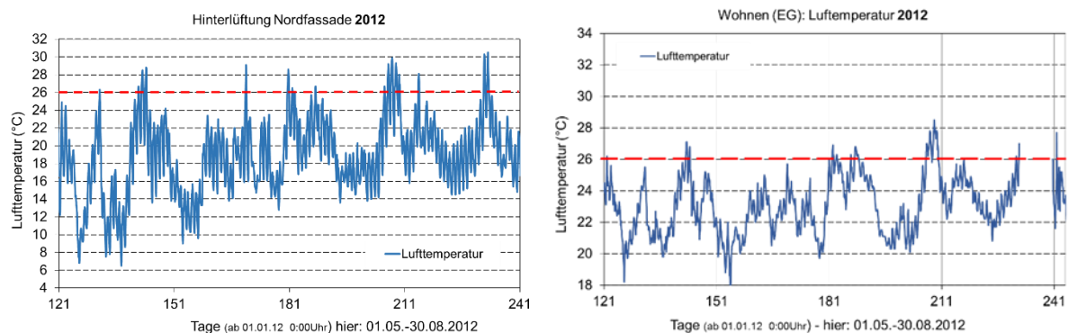
BILD 7-9 GEMESSENE RAUMLÜFTTEMPERATUREN IM WOHNRAUM UND ZUGEORDNETE AUßENLÜFTTEMPERATUREN IN DER HINTERLÜFTUNGSEBENE DER NNO-WAND VOM 1. MAI BIS 30. AUGUST 2012
