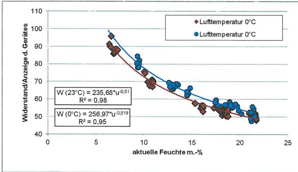
BILD 9-14 EXPERIMENTELL ERMITTELTE BEZIEHUNG ZWISCHEN DEM ELEKTRISCHEN WIDERSTAND UND DER MATERIALFEUCHTE AN FURNIERSCHICHTHOLZ (KERTO) LÄNGS ZUR FASER BEI TEMPERATUREN VON 23°C UND VON 0°C
