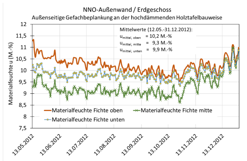
BILD 7-41 MESSWERTE ZUR MATERIALFEUCHTE IN DER AUßENSEITIGEN OSB-GEFACHBEPLANKUNG DER NNO-AUßENWAND (EG) VON 2012
