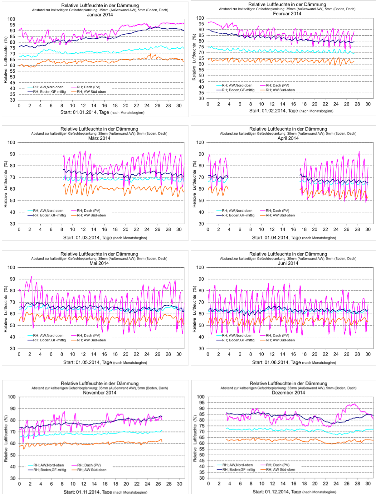
BILD 9-53 RELATIVE LUFTFEUCHTEN IN DER GEFACHDÄMMUNG DER AUßENWAND, DER BODENPATTE UND DES DACHES VON JANUAR BIS JUNI 2014 UND VON NOVEMBER BIS DEZEMBER 2014
