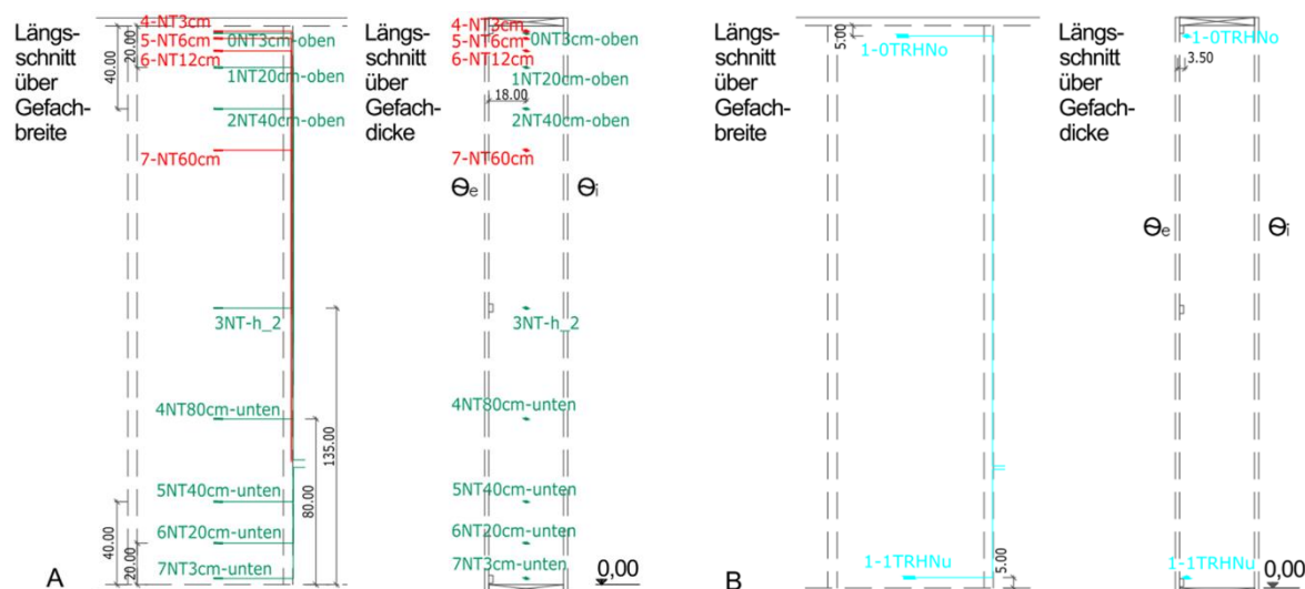
BILD 6-2 ÜBERSICHTSZEICHNUNGEN A) ZUR ANORDNUNG VON TEMPERATURFÜHLERN IN DER GEFACHDÄMMUNG UND B) ZUR ANORDNUNG VON FÜHLERN ZUR MESSUNG DER RELATIVEN LUFTFEUCHTE UND DER TEMPERATUR IN DER GEFACHDÄMMUNG
