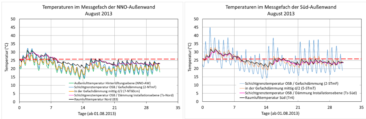
BILD 7-22 GEMESSENE TEMPERATUREN ÜBER DEN QUERSCHNITT DER NNO- UND SSW-AUßENWAND IM AUGUST 2013
