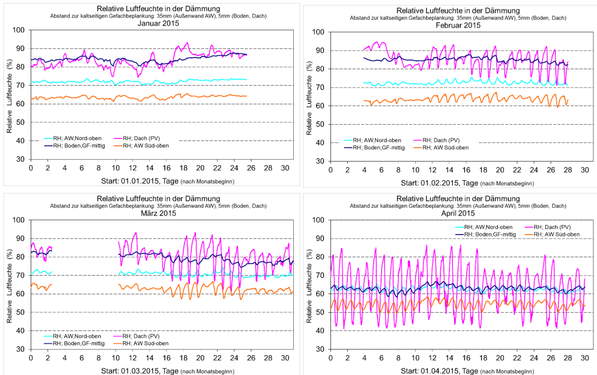
BILD 9-54 RELATIVE LUFTFEUCHTEN IN DER GEFACHDÄMMUNG DER AUßENWAND, DER BODENPATTE UND DES DACHES VON JANUAR BIS APRIL 2015
