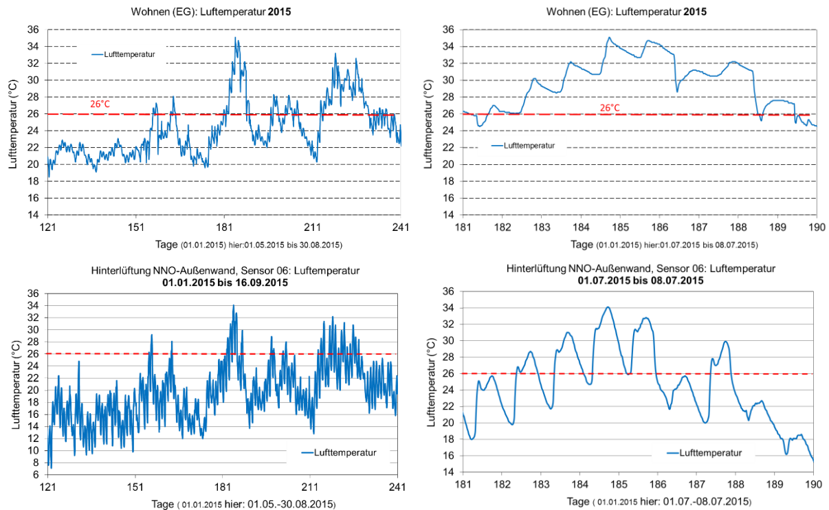
BILD 7-13 GEMESSENE RAUMLUFTTEMPERATUREN IM WOHNRAUM SOWIE GEMESSENE AUßENLUFTTEMPERATUREN IN DER HINTERLÜFTUNGSEBENE DER NNO-AUßENWAND FÜR 2015: VOM 01. 05.-31.08. UND VOM 01.07.-08.07.2015
