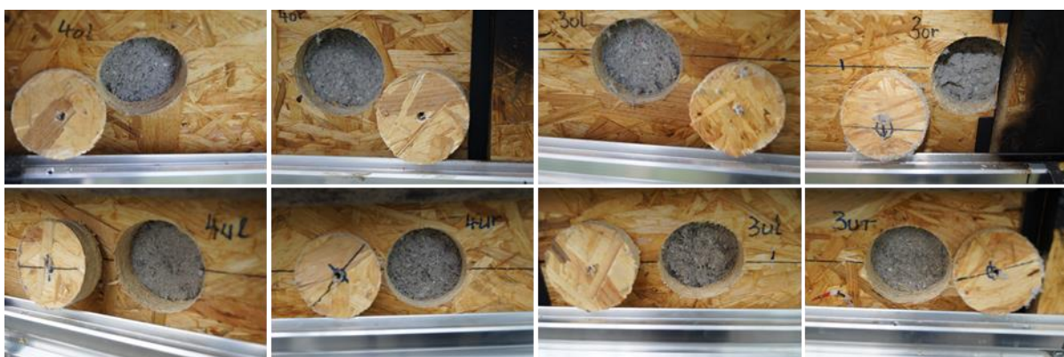
BILD 9-17 ZUSTAND DER SCHICHTGRENZE GEFACHDÄMMUNG / AUßENSEITIGE GEFACHBEPLANKUNG AN GEFACH 3 UND 4 AM 27.04.2012
