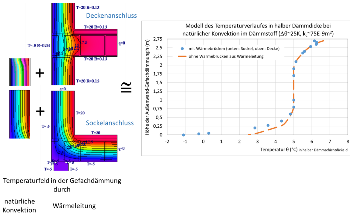
BILD 5-2 VEREINFACHTES TEMPERATURFELD-MODELL FÜR DIE AUßENWAND-GEFACHDÄMMUNG MIT DEN SICH ÜBERLAGERNDEN WÄRMETRANSPORTANTEILEN WÄRMELEITUNG UND NATÜRLICHE KONVEKTION
