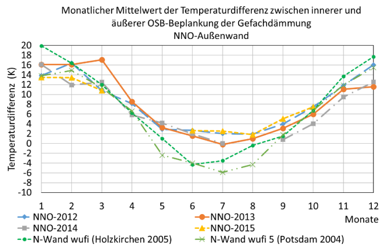
BILD 7-17 MONATLICHE MITTELWERTE DER TEMPERATURDIFFERENZEN ZWISCHEN INNEN- UND AUßENSEITIGER OSB-BEPLANKUNG DER GEFACHDÄMMUNG VON 2012 BIS 2015, FÜR DIE NNO-AUßENWAND
