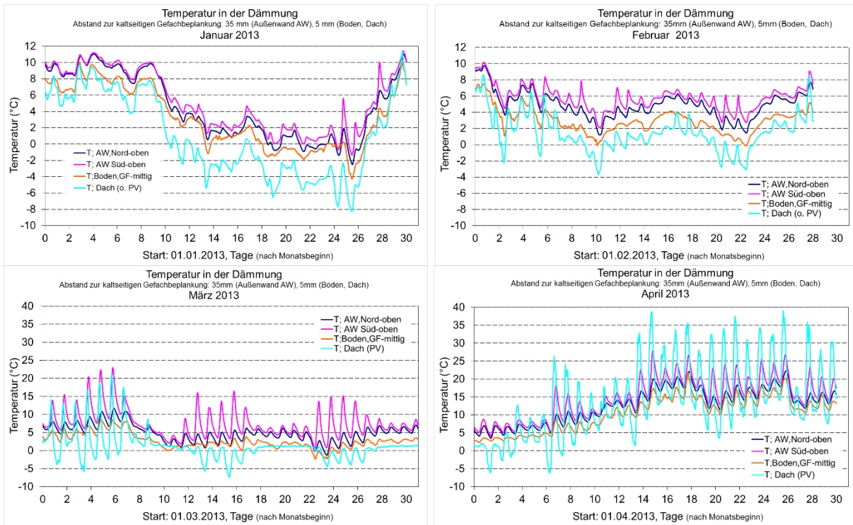
BILD 9-56 TEMPERATUR IN DER GEFACHDÄMMUNG DER ÄUßENWAND, DER BODENPATTE UND DES DACHES VON JANUAR 2013 BIS APRIL 2013 (ZUZUORDNEN DER RELATIVEN LUFTFEUCHTE AUS ABSCHNITT 9.4.3)
