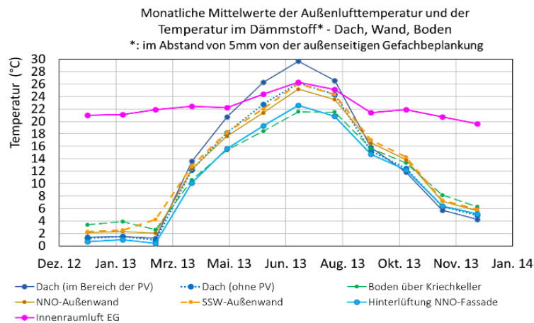
BILD 7-38 MONATLICHE MITTELWERTE DER GEMESSENEN TEMPERATUREN INNERHALB DER GEFACHDÄMMUNG DER AUßENBAUTEILE AUßENWAND, BODEN UND DACH MIT 5MM ABSTAND ZUR AUßENSEITIGEN GEFACHBEPLANKUNG FÜR 2013
