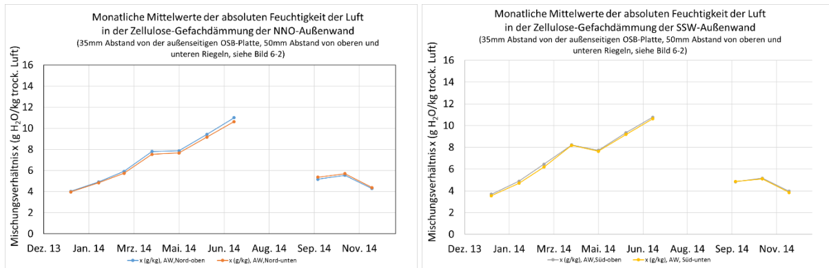
BILD 7-49 GEMESSENE MONATLICHE MITTELWERTE DER ABSOLUTEN FEUCHTIGKEIT DER LUFT IM DÄMMSTOFF IM ABSTAND VON 35MM VON DER AUßENSEITIGEN GEFACHBEPLANKUNG DER NNO-AUßENWAND UND DER SSW-AUßENWAND FÜR 2014
