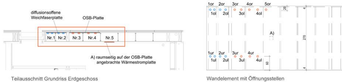
BILD 6-1 ÜBERSICHTSZEICHNUNG ZUR ANORDNUNG VON „ENTNAHMESTELLEN“ IN DEN AUßENSEITIGEN GEFACHBEPLANKUNGEN IN DER NNO-AUßENWAND DES ERDGESCHOSSES
