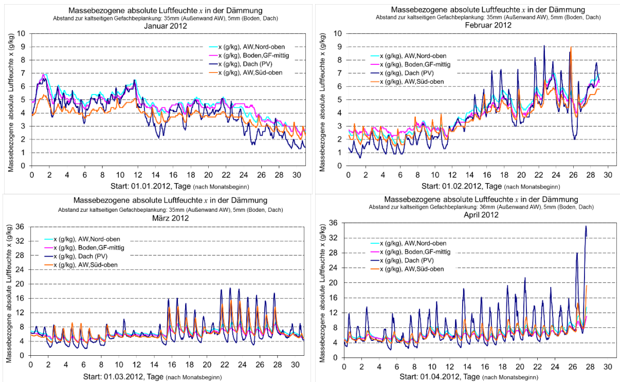
BILD 9-59 MASSEBEZOGENE ABSOLUTE LUFTFEUCHTE IN DER GEFACHDÄMMUNG DER AUßENWAND, DER BODENPATTE UND DES DACHES VON JANUAR 2012 BIS APRIL 2012
