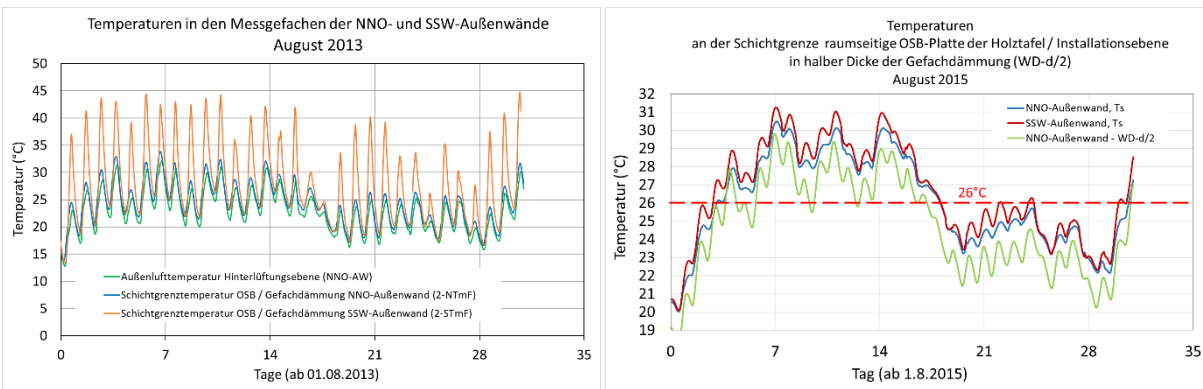
BILD 7-27 GEMESSENE TEMPERATUREN INNERHALB DER NNO-AUßENWAND UND DER SSW-AUßENWAND IM AUGUST 2013 UND 2015
