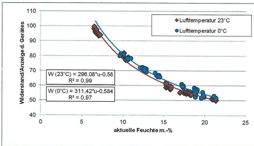
BILD 9-13 EXPERIMENTELL ERMITTELTE BEZIEHUNG ZWISCHEN DEM ELEKTRISCHEN WIDERSTAND UND DER MATERIALFEUCHTE AN FURNIERSCHICHTHOLZ (KERTO) QUER ZUR FASER BEI TEMPERATUREN VON 23°C UND VON 0°C
