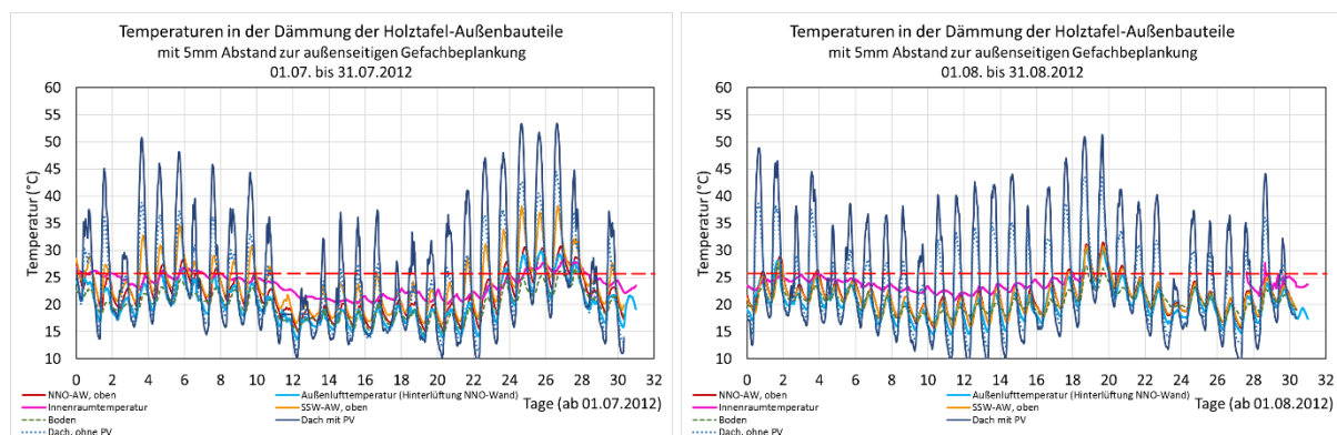
BILD 7-28 GEMESSENE TEMPERATUREN NAHE DEN SCHICHTGRENZEN DER AUßENSEITIGEN OSB-PLATTEN DER NNO- UND SSW-AUßENWAND, DER BODENPLATTE (ÜBER DEM KRIECHKELLER: ZEMENTGEBUNDENE SPANPLATTE) UND IM DACH IM JULI 2015
