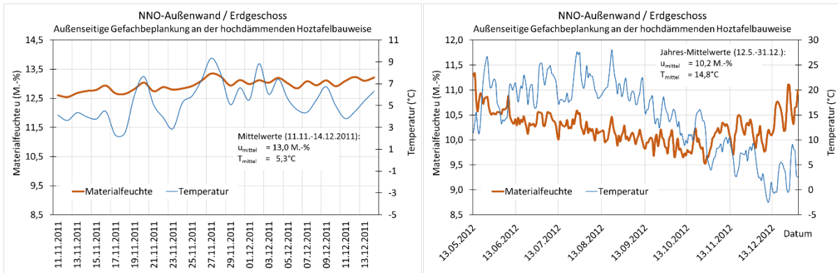
BILD 9-32 GEMESSENE MATERIALFEUCHTEN UND TEMPERATUREN ALS TÄGLICHE MITTELWERTE IN DER AUßENSEITIGEN GEFACHBEPLANKUNG DER NNO-AUßENWAND / ERDGESCHOSS FÜR DEZEMBER 2011 (EINBAU) UND FÜR 2012
