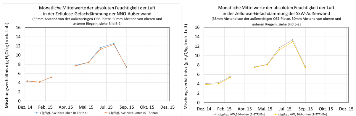
BILD 7-50 GEMESSENE MONATLICHE MITTELWERTE DER ABSOLUTEN FEUCHTIGKEIT DER LUFT IM DÄMMSTOFF IM ABSTAND VON 35MM VON DER AUßENSEITIGEN GEFACHBEPLANKUNG DER NNO-AUßENWAND UND DER SSW-AUßENWAND FÜR 2015
