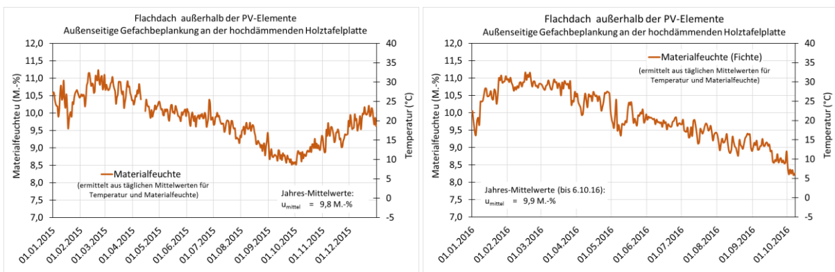
BILD 9-43 GEMESSENE MATERIALFEUCHTEN UND TEMPERATUREN ALS TÄGLICHE MITTELWERTE IN DER AUßENSEITIGEN GEFACHBEPLANKUNG DER HOLZTAFELPLATTE DES FLACHDACHES AUßERHALB DER PV-ELEMENTE FÜR 2015 UND 1.1.-06.10. 2016
