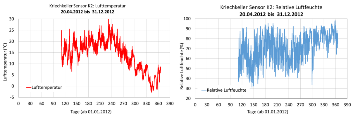
BILD 7-5 GEMESSENE TEMPERATUREN UND RELATIVE LUFTFEUCHTEN IM KRIECHKELLER VOM 20.04.2012 BIS 31.12.2012
