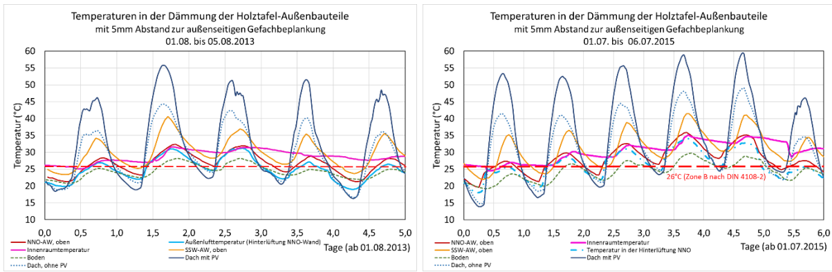
BILD 7-31 TEMPERATUREN INNERHALB DER GEFACHDÄMMUNG DER AUßENBAUTEILE, GEMESSEN IM ABSTAND VON 5MM ZUR AUßENSEITIGEN GEFACHBEPLANKUNG: 1.-5. AUGUST 2013 UND VOM 1.-7. JULI 2015
