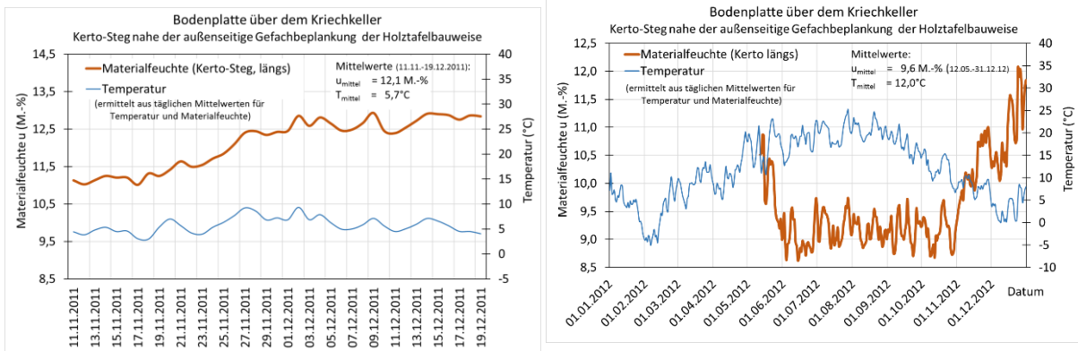
BILD 9-47 GEMESSENE MATERIALFEUCHTEN UND TEMPERATUREN ALS TÄGLICHE MITTELWERTE AN DER AUßENSEITIGEN GEFACHBEPLANKUNG DER HOLZTAFELPLATTE DER BODENPLATTE ÜBER DEM KRIECHKELLER FÜR DEZEMBER 2011 (EINBAU) UND FÜR 2012, MESSWERTE DER SENSOREN 7-BFK1 UND 8-BTK-SW
