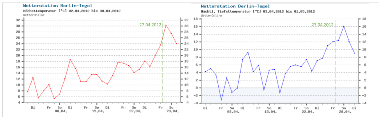
BILD 9-19 HÖCHST- UND TIEFSTTEMPERATUREN VOR UND WÄHREND DER ORTSBESICHTIGUNG AM 27.04.2012 (QUELLE: WWW.WETTERONLINE.DE)
