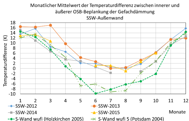
BILD 7-18 MONATLICHE MITTELWERTE DER TEMPERATURDIFFERENZEN ZWISCHEN INNEN- UND AUßENSEITIGER OSB-BEPLANKUNG DER GEFACHDÄMMUNG VON 2012 BIS 2015, FÜR DIE SSW-AUßENWAND
