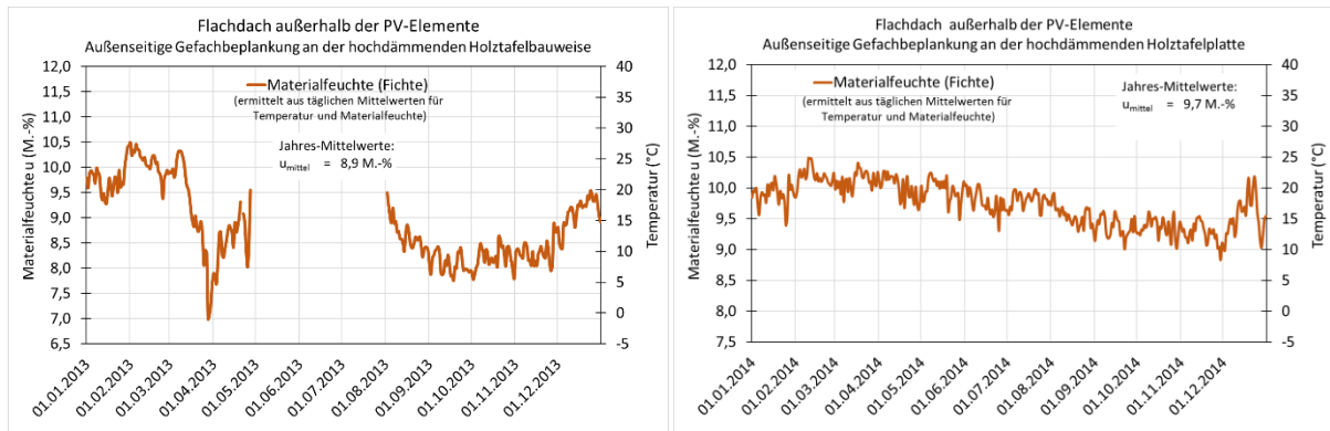
BILD 9-42 GEMESSENE MATERIALFEUCHTEN UND TEMPERATUREN ALS TÄGLICHE MITTELWERTE IN DER AUßENSEITIGEN GEFACHBEPLANKUNG DER HOLZTAFELPLATTE DES FLACHDACHES AUßERHALB DER PV-ELEMENTE FÜR 2013 UND 2014
