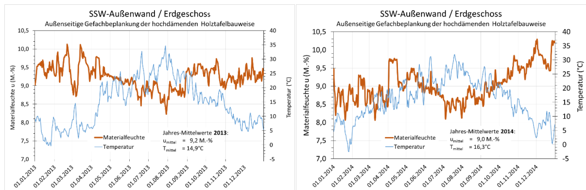
BILD 9-36 GEMESSENE MATERIALFEUCHTEN UND TEMPERATUREN ALS TÄGLICHE MITTELWERTE IN DER AUßENSEITIGEN GEFACHBEPLANKUNG DER SSW-AUßENWAND / ERDGESCHOSS FÜR 2013 UND 2014
