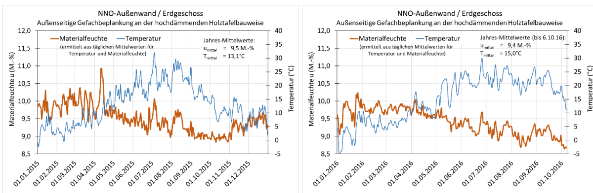
BILD 9-34 GEMESSENE MATERIALFEUCHTEN UND TEMPERATUREN ALS TÄGLICHE MITTELWERTE IN DER AUßENSEITIGEN GEFACHBEPLANKUNG DER NNO-AUßENWAND / ERDGESCHOSS FÜR 2015 UND VOM 1.1.-06.10. 2016
