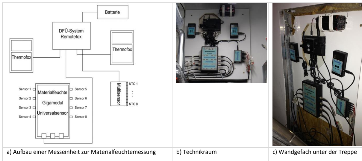
BILD 6-5 PRINZIPISSKIZZE UND FOTOS ZUM AUFBAU EINER MESSEINHEIT ZUR DATENERFASSUNG, DATENSPEICHERUNG UND DATENFERNÜBERTRAGUNG FÜR 8 MATERIALFEUCHTEMESSTELLEN UND 8 NTC-TEMPERATURFÜHLER
