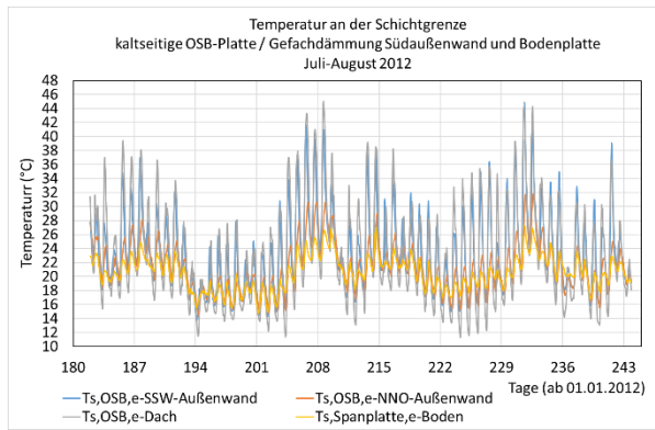
BILD 7-33 GEMESSENE TEMPERATUREN AN DER SCHICHTGRENZE DER AUßENSEITIGEN GEFACHBEPLANKUNG DER NNO-AUßENWAND, SSW-AUßENWAND, IM DACH (AUßERHALB DES BEREICHES DER PV-ELEMENTE) UND IN DER BODENPLATTE ÜBER DEM KRIECKELLER VON JULI BIS AUGUST 2012
