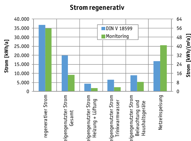
Abbildung 25: Vergleich von Simulation und Messung der Stromerzeugung
